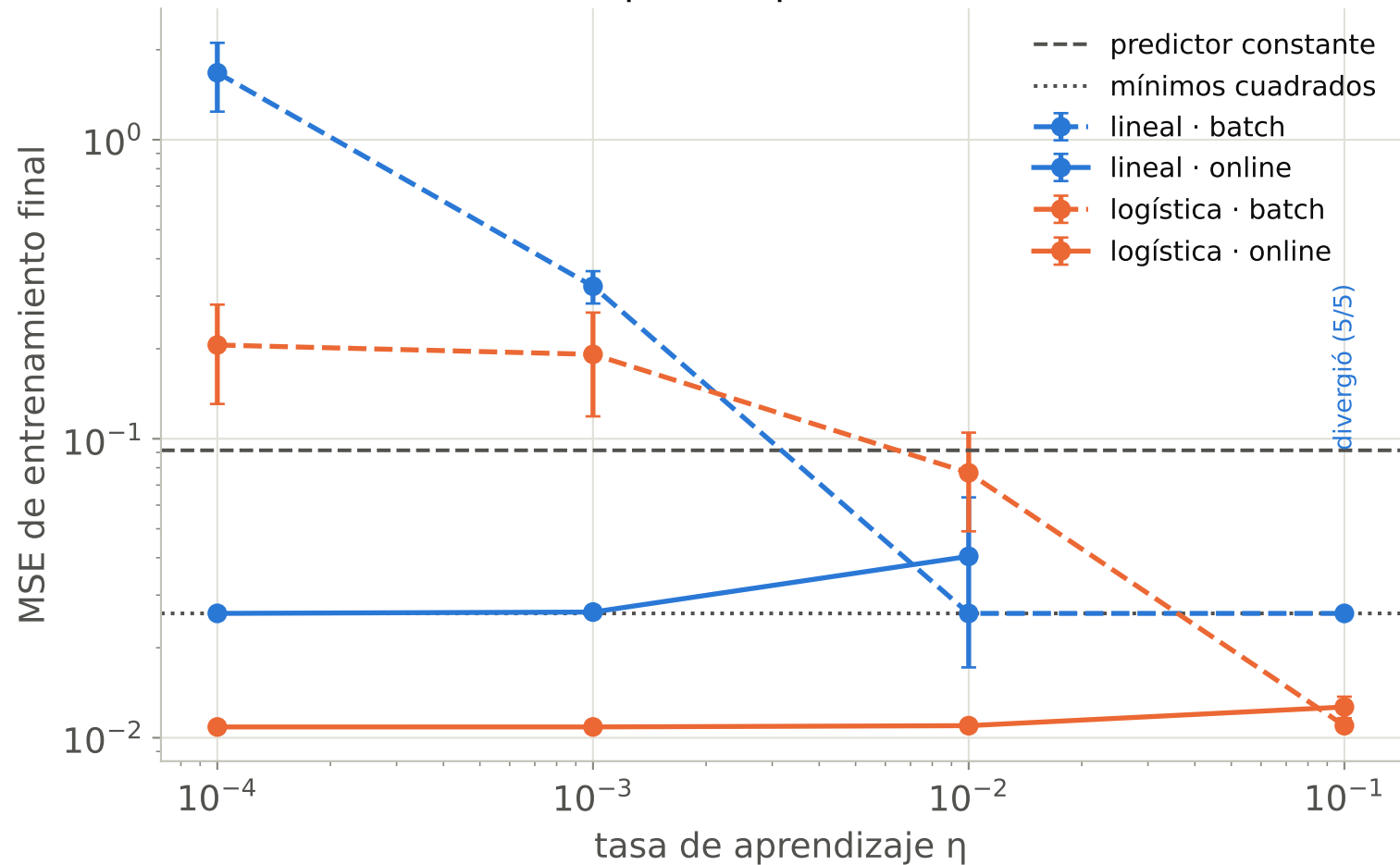
Sensibilidad a \eta (500 épocas, media \pm desvío)
