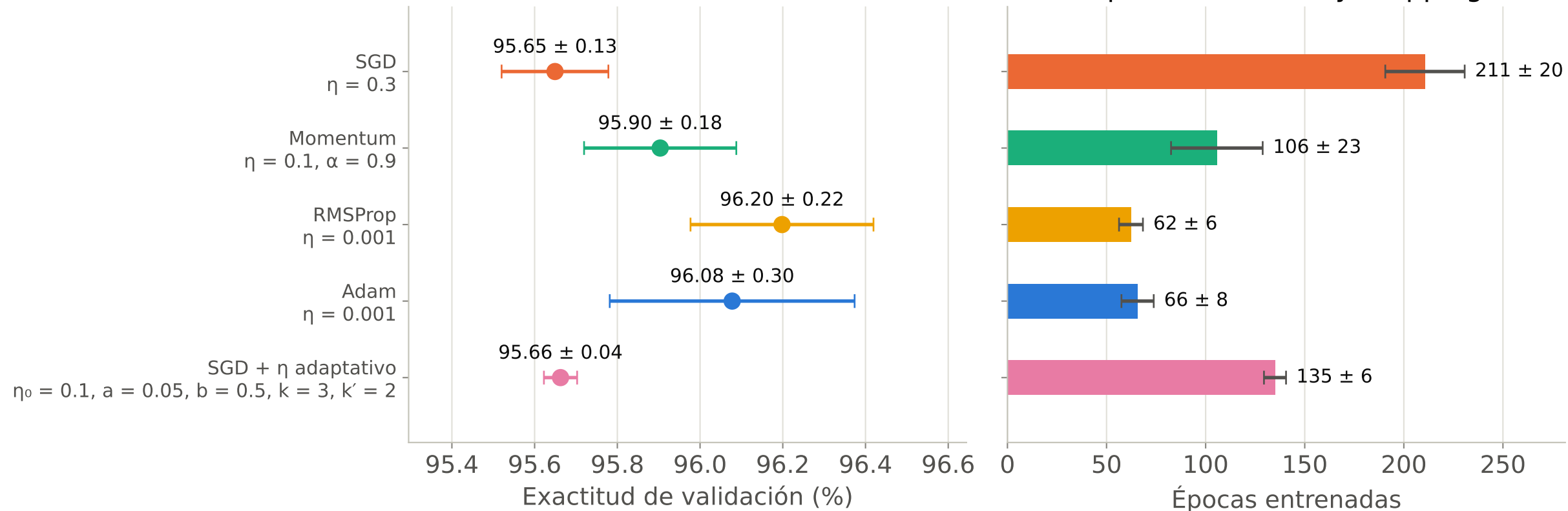
Épocas hasta Early Stopping
