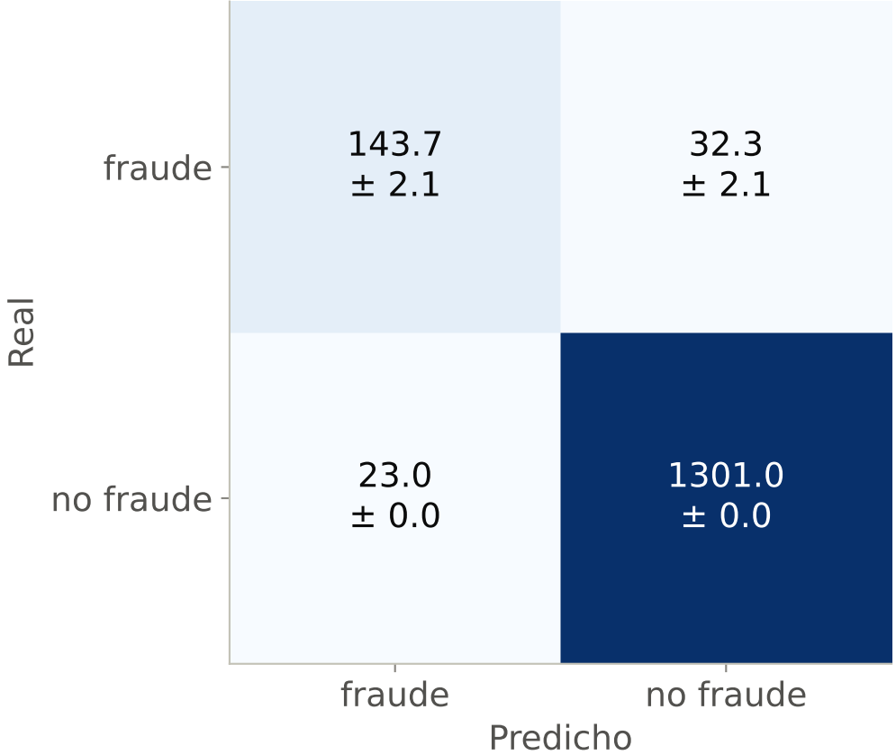
Matriz de confusión (media de 3 modelos)
