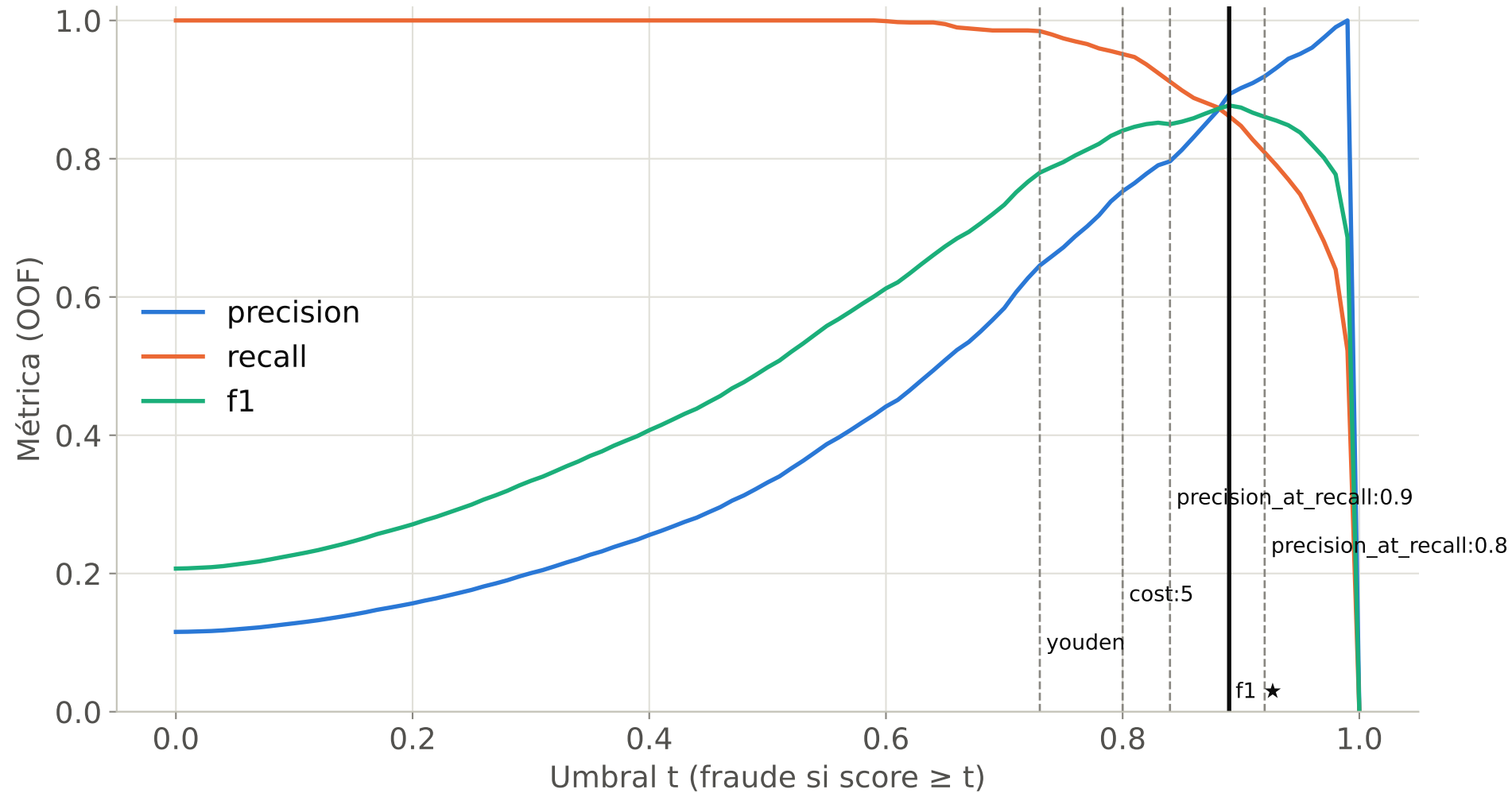
E1-B-c · Métricas vs umbral (OOF), umbrales de cada criterio (★ recomendado)
