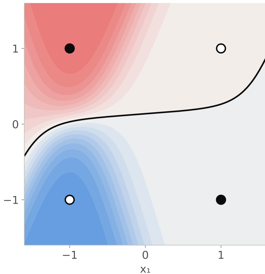
MLP [2, 2, 1], peor semilla semilla 12: no resuelve
