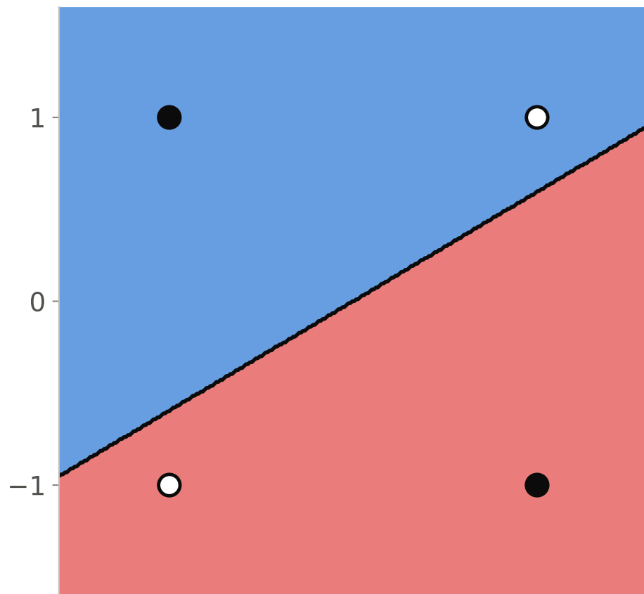
escalón [2, 1] semilla 0: no resuelve
