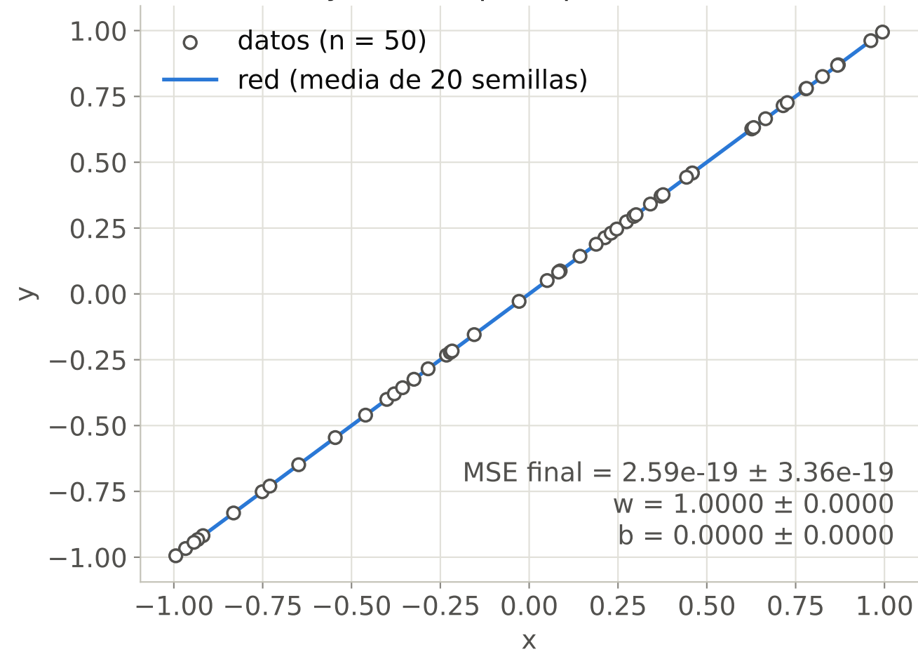
y = x con perceptrón lineal
