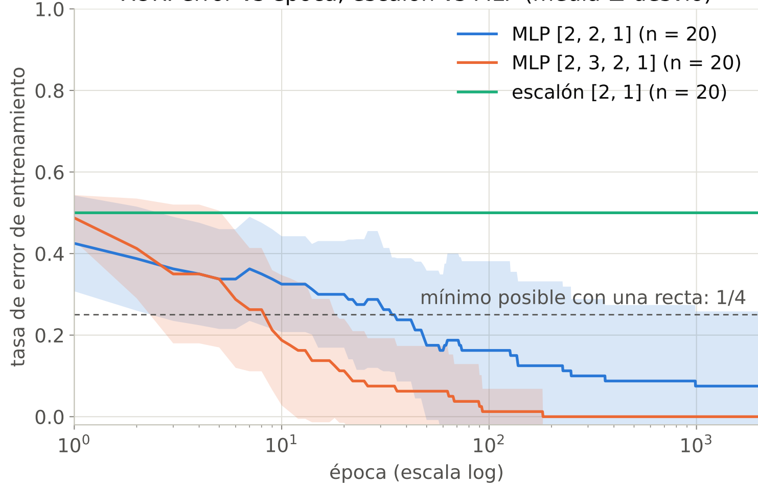
XOR: error vs época, escalón vs MLP (media \pm desvío)
