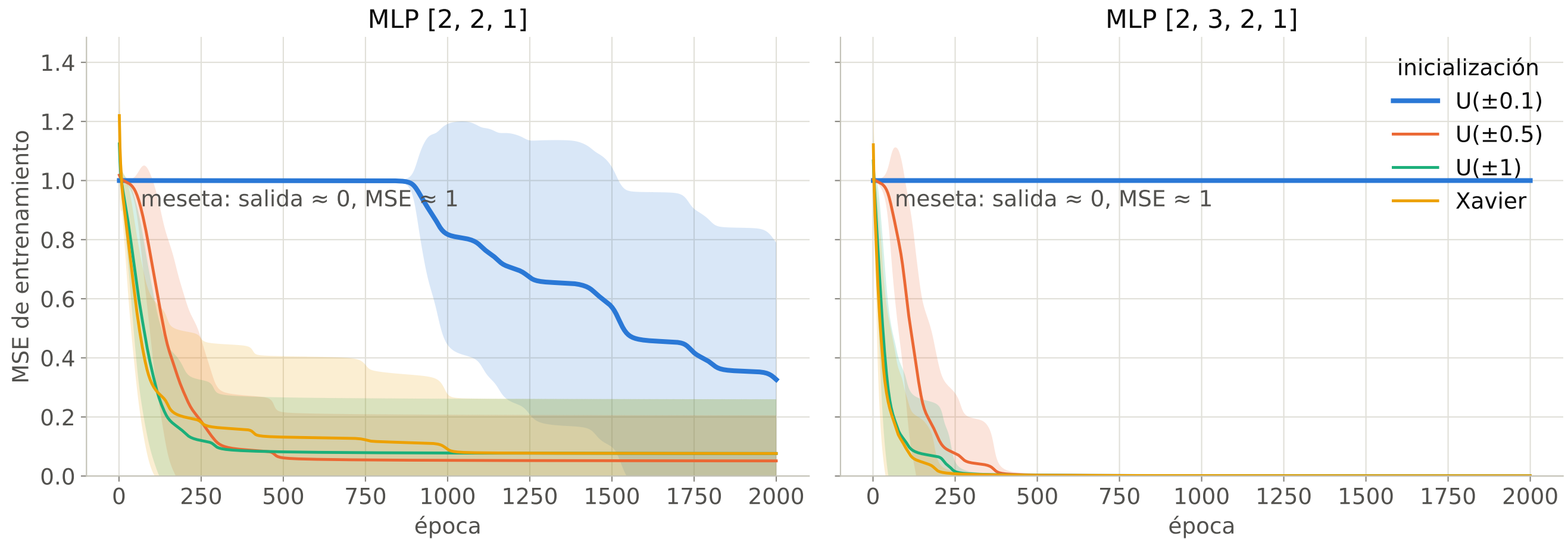
XOR: loss vs época según la inicialización ( \eta = 0.1 , media \pm desvío, n = 20 semillas)
