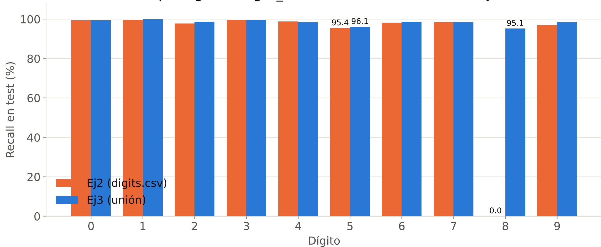
Recall por dígito en digits_test.csv · modelo final de cada ejercicio
