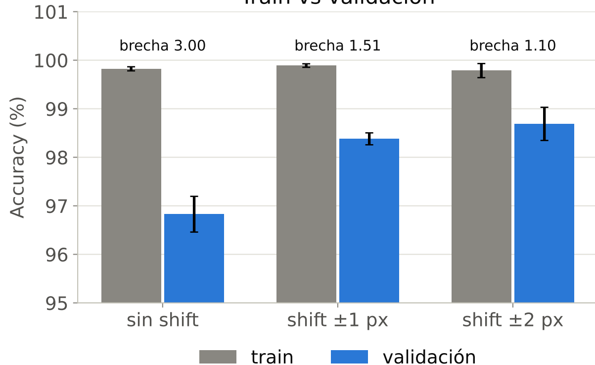
Train vs validación
