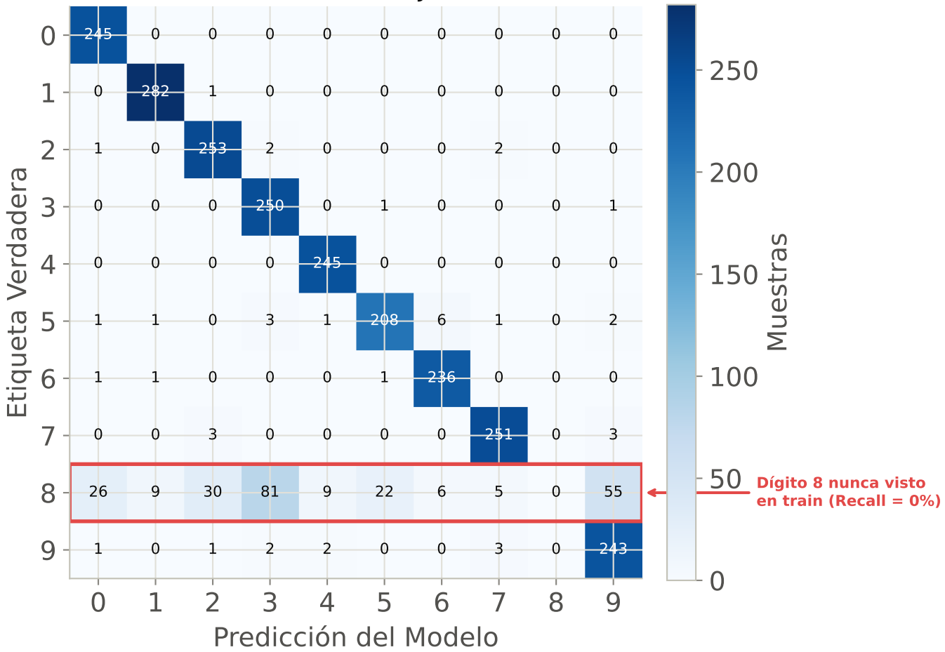
Matriz de Confusión en Test (Ej2 Final, Acc=88.31%)
