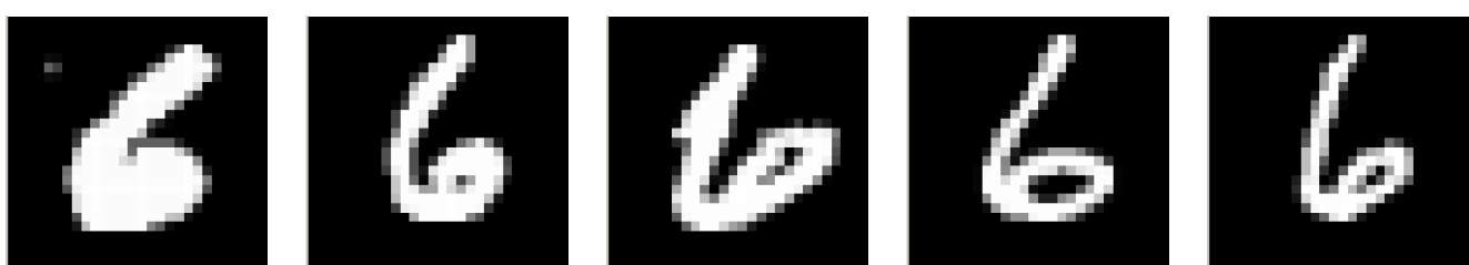
Dígito 6
