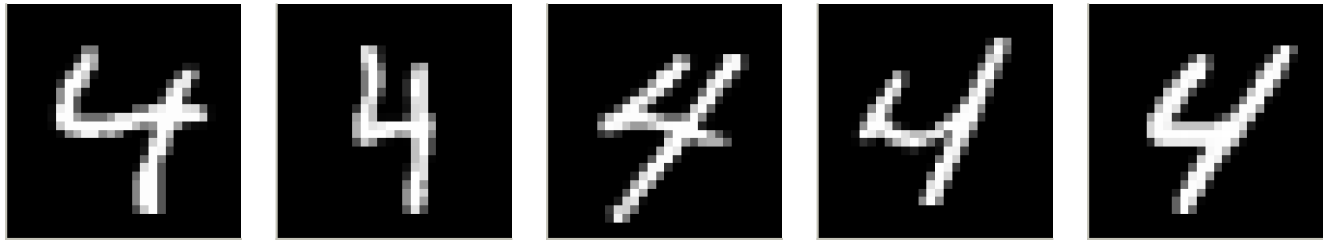
Dígito 4
