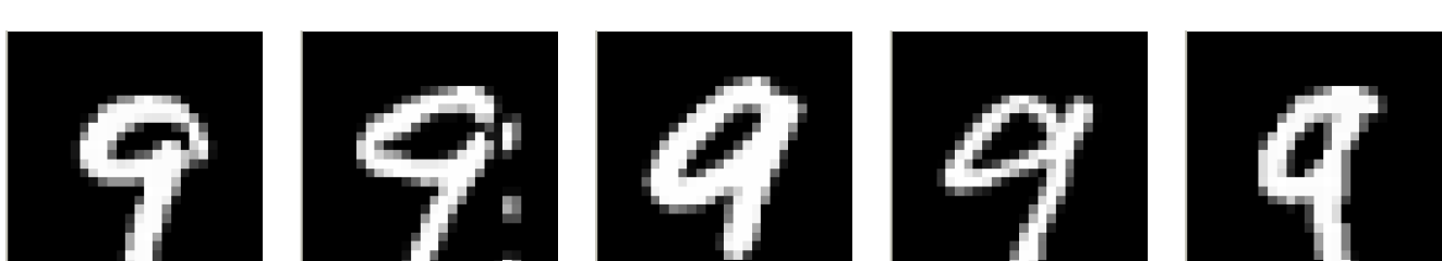
Dígito 9
