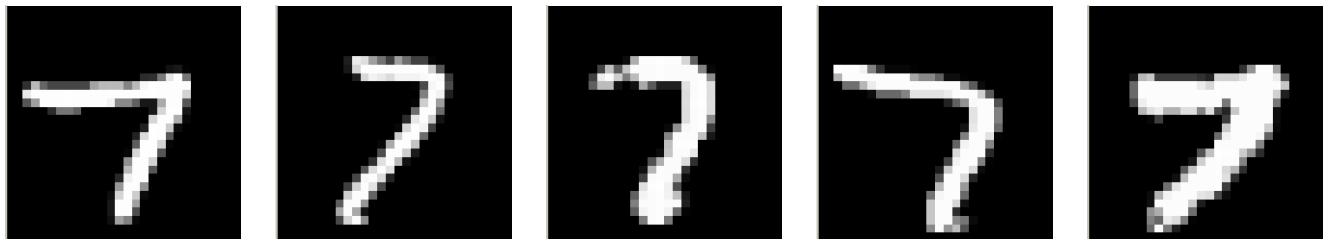
Dígito 7
