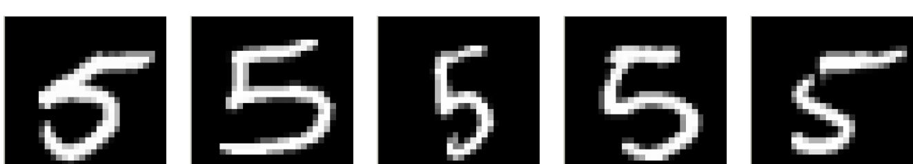
Dígito 5
