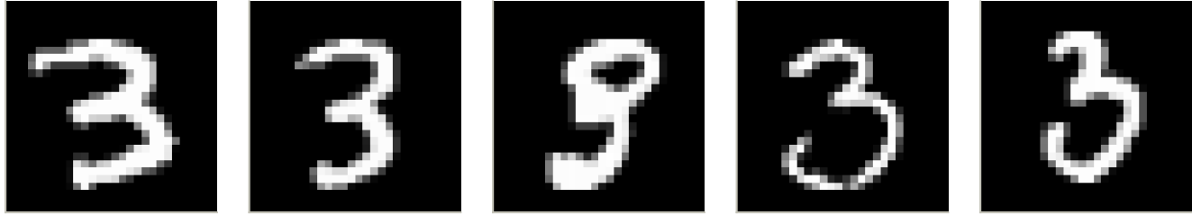
Dígito 3
