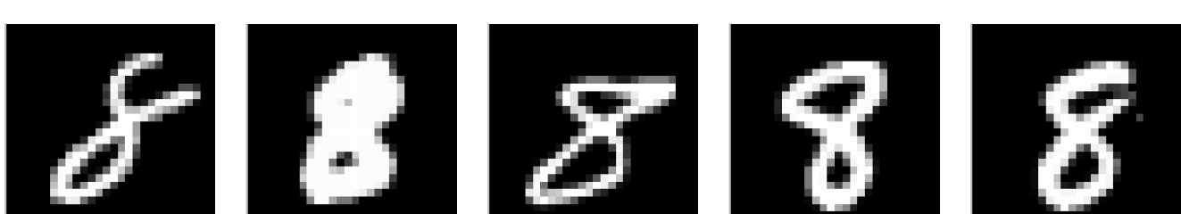
Dígito 8 (test)
