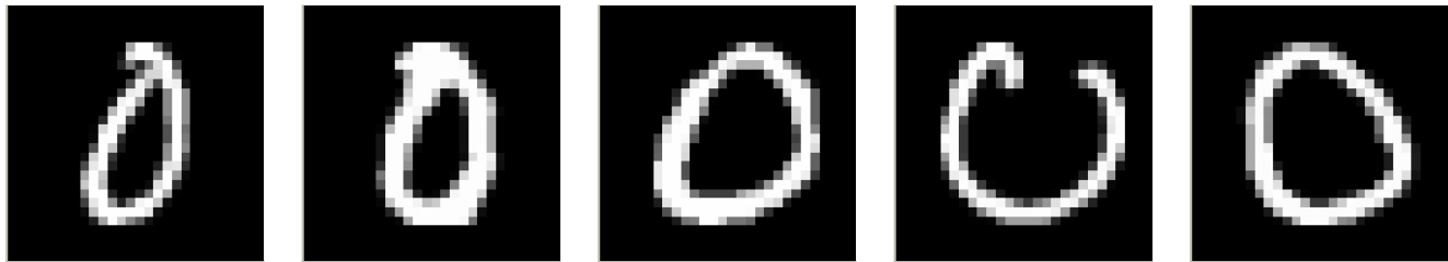
Dígito 0
