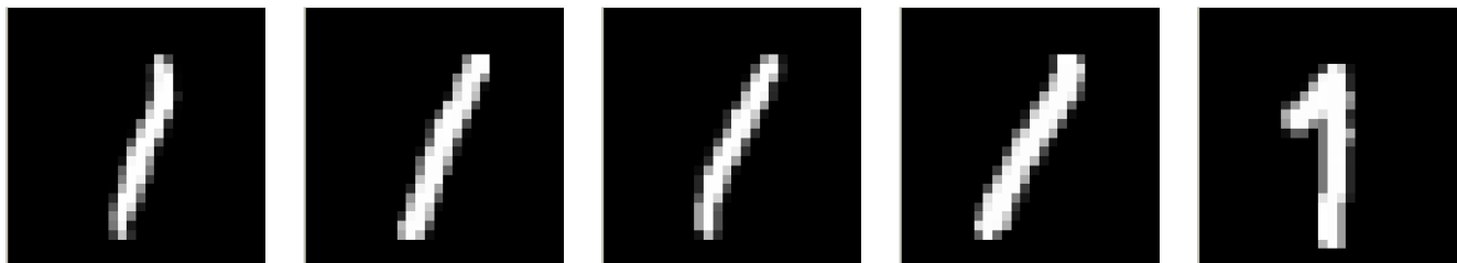
Dígito 1
