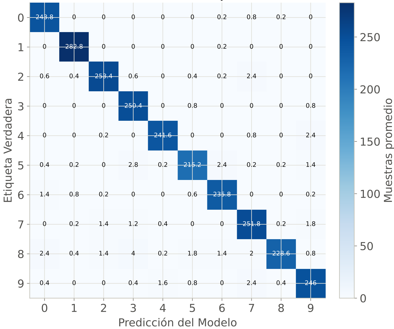
Matriz de Confusión Oficial en Test (Ej3 Final, Acc = 98.09%)
