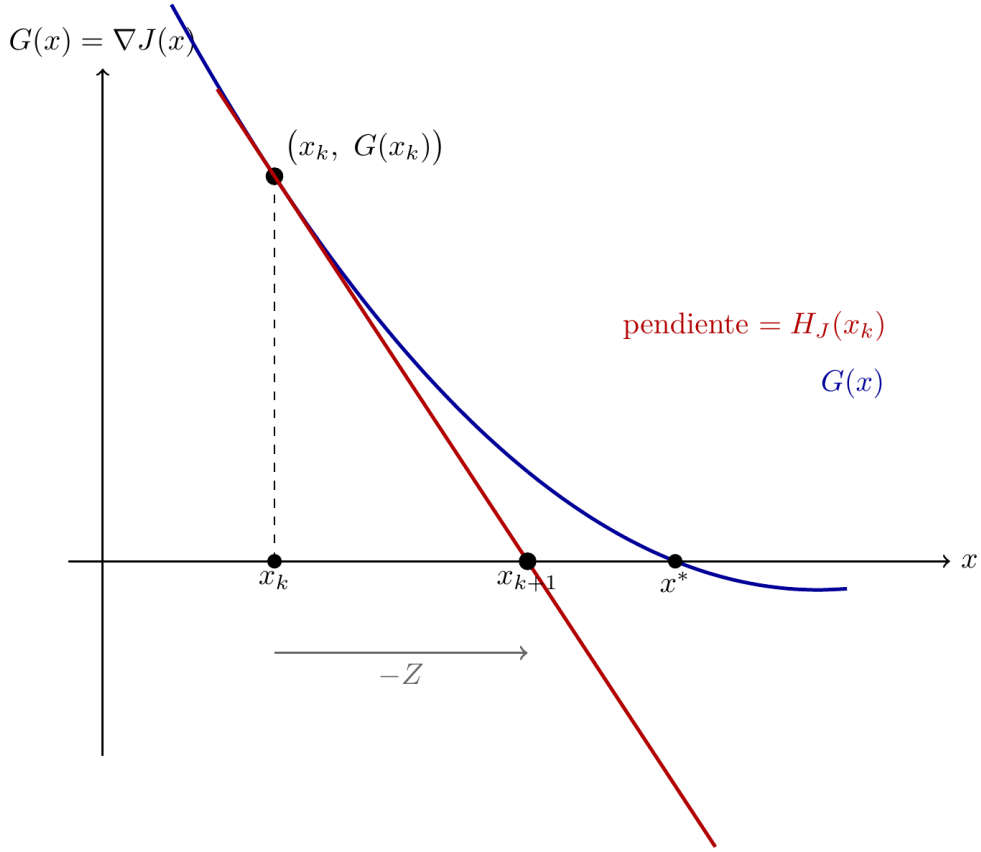
Figura 3.1: Descripción geométrica del método de Newton.
