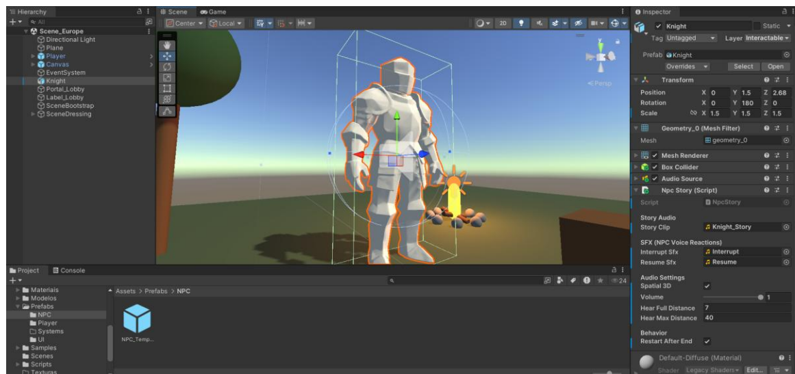
Figura 5. Screenshot da janela Hierarchy do Unity Editor, mostrando a estrutura wrapper prefab aplicada a um dos NPCs. Ao lado, o painel Inspector destacando os componentes anexados ao GameObject raiz.
