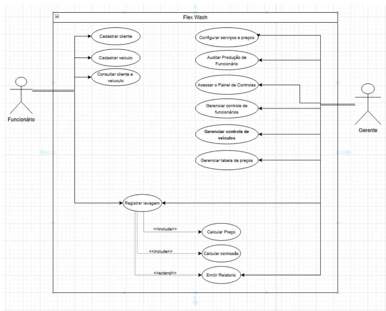
Figura 1 - Diagrama UML
