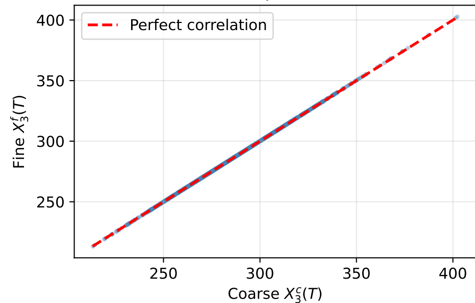
Asset 3: \rho = 1.0000
