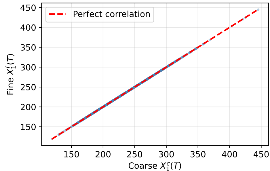
Asset 1: \rho = 1.0000
