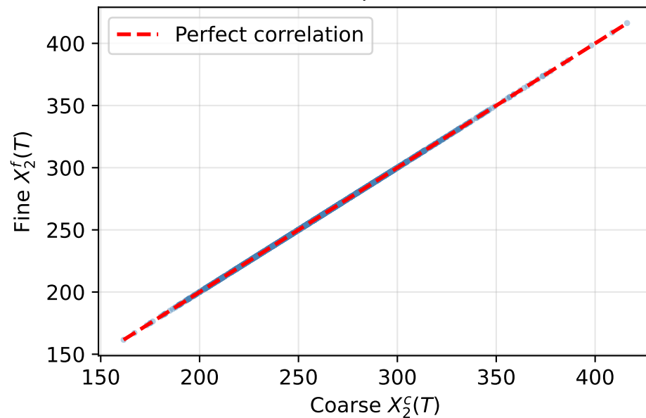
Asset 2: \rho = 1.0000
