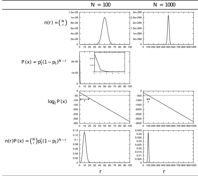
Figura 18: Considerando p = 0,1 , n = 100 e n = 1000 os gráficos ilustram n(r) , o número de strings contendo r 1s; a probabilidade Pr(x_{1:n}) para uma sequência contendo r 1s; a mesma probabilidade em escala logarítmica; e a probabilidade total n(r)Pr(x_{1:n}) de todas as sequências contendo r 1s (MacKay 2003).
