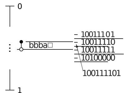
Figura 41: Definição dos intervalos probabilísticos para uma sequência binária na saída do codificador (MacKay 2003).
