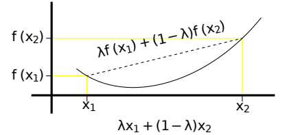
Figura 11: Ilustração de uma função convexa no intervalo.
