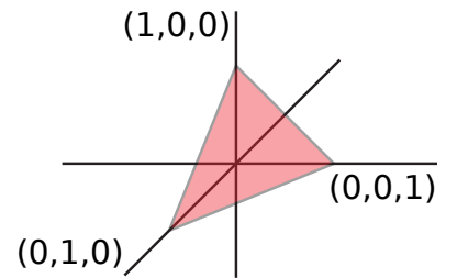
Figura 20: Simplex probabilístico para m = 2 .
