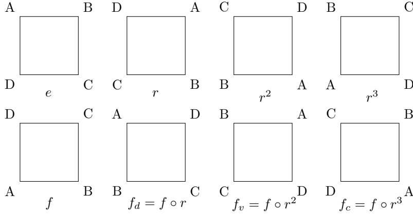
Figura 56: As oito simetrias do quadrado, geradas pelos elementos r (rotação de 90 graus no sentido horário) e f (reflexão vertical), sob a operação de composição.
