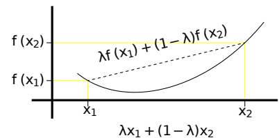
Figura 11: Ilustração de uma função convexa no intervalo.
