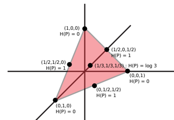
Figura 23: Simplex probabilístico para m = 3 .
