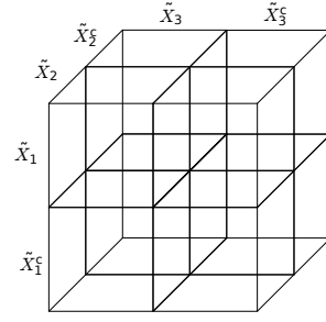
Figura 14: Exemplo de átomos para n = 3 .
