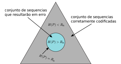
Figura 25: Representação das sequências em um simplex probabilístico. As sequências com H(P_{x_{1:n}}) \leq R_n não acarretarão em erro no processo de codificação.
