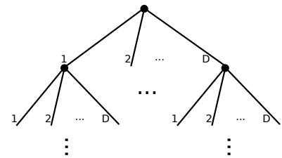
Figura 32: Árvore D -ária.
