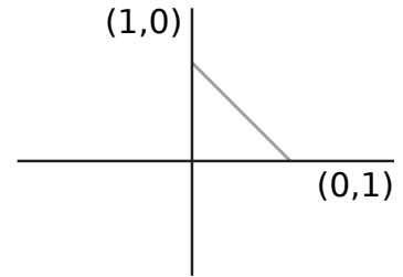
Figura 22: Simplex probabilístico para m = 2 .
