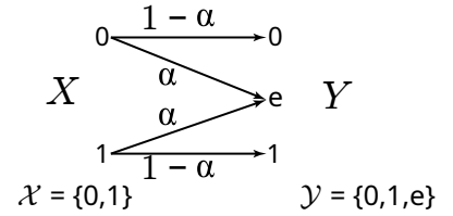
Figura 53: Canal binário com apagamento.
