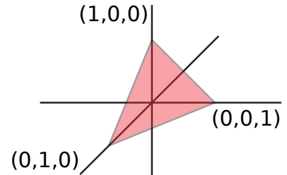
Figura 22: Simplex probabilístico para m = 2 .
