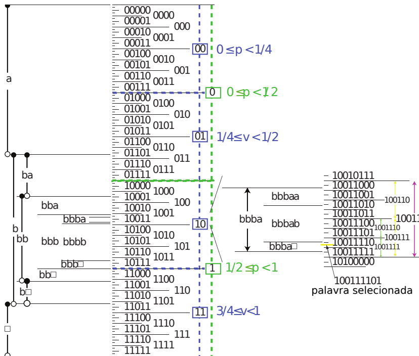
Figura 42: Todo o processo de subdivisão dos intervalos para a sequência de símbolos da fonte e para a sequência binária na saída do codificador (MacKay 2003).
