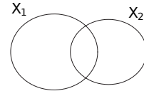
Figura 15: Diagrama de informação para X_1 e X_2 .
