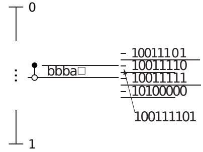
Figura 41: Intervalo final para a sequência de símbolos da fonte e para a sequência binária na saída do codificador.
