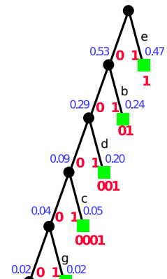
Figura 33: Árvore obtida através do método guloso seguindo a estratégia top-down .
