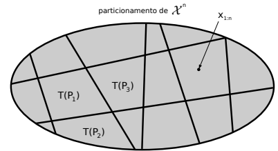
Figura 20: Particionamento do espaço de sequências de comprimento n .
