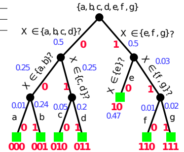
Figura 33: Árvore obtida através do método guloso seguindo a estratégia top-down .
