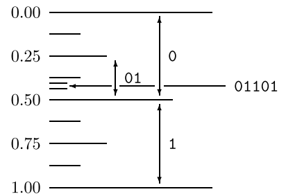
Figura 39: Definição dos intervalos probabilísticos para uma sequência de símbolos produzida pela fonte.
