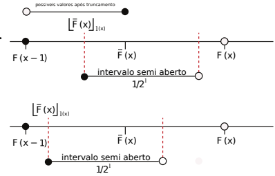
Figura 38: Intervalo de comprimento 1/2^l representando [\overline{F}(x)]_{l(x)} como uma forma não ambígua para codificação.
