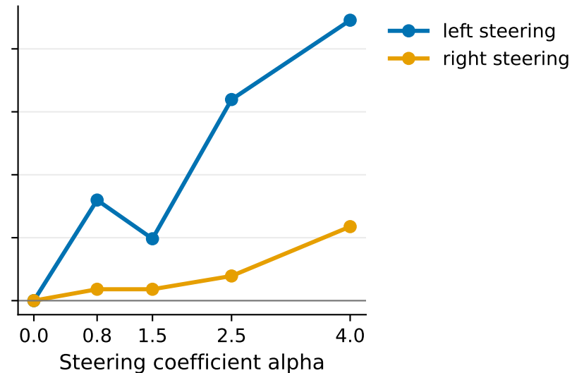
Llama-3
