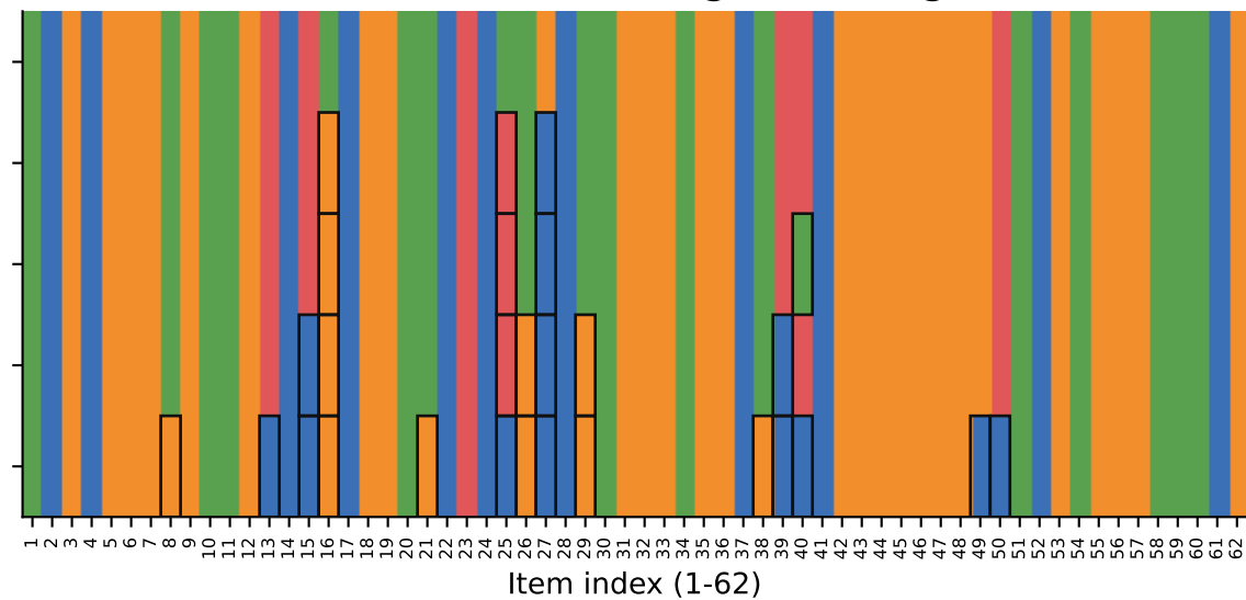
Llama-3 German: right steering
