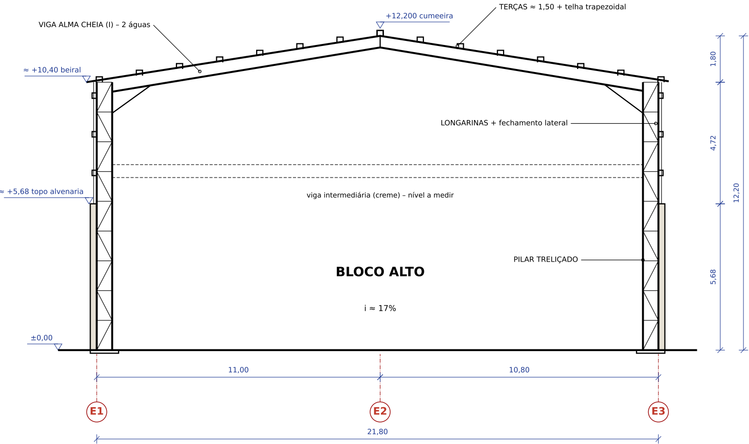
CORTE C-C - BLOCO ALTO (transversal)
