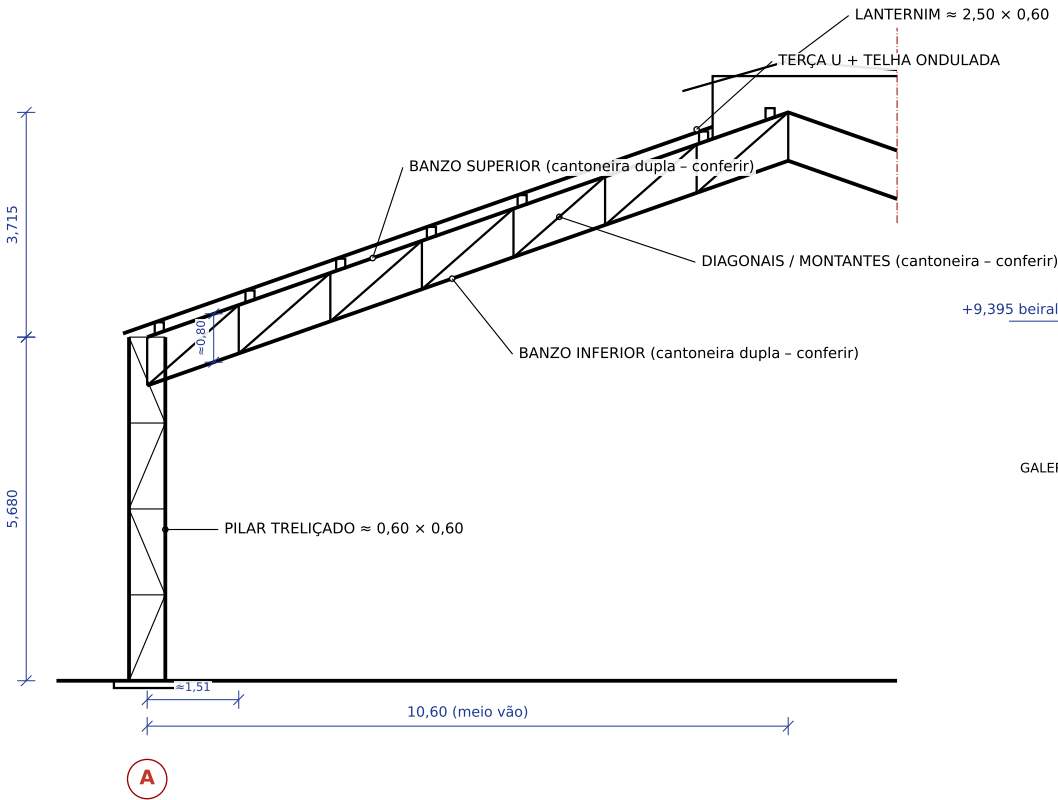
DETALHE 1 - TRELIÇA TÍPICA E LANTERNIM (Nave 1)
