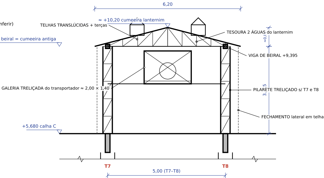
CORTE B-B - LANTERNIM ELEVADO (na calha C)
