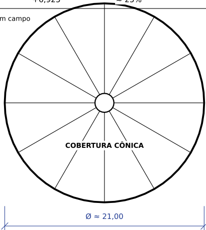
D7 - SILO METÁLICO
