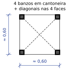
DET. 2 - PILAR
