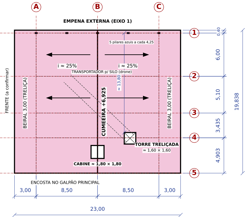
D1 - MOEGA 3 (campo + drone)
