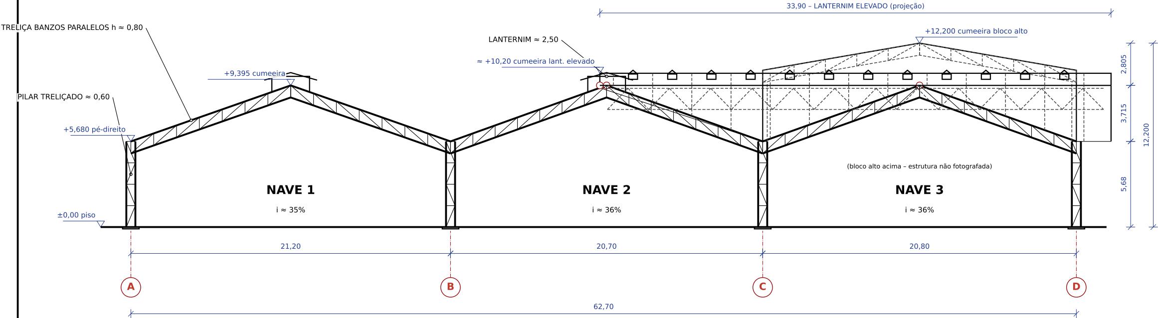
CORTE A-A - GALPÃO PRINCIPAL (transversal)
