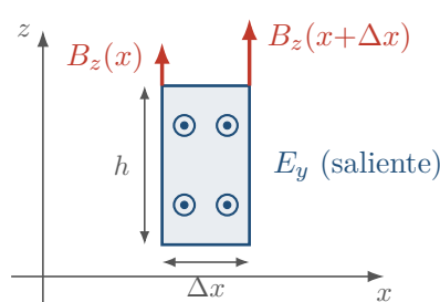
(b) plano xz : Ampère–Maxwell
