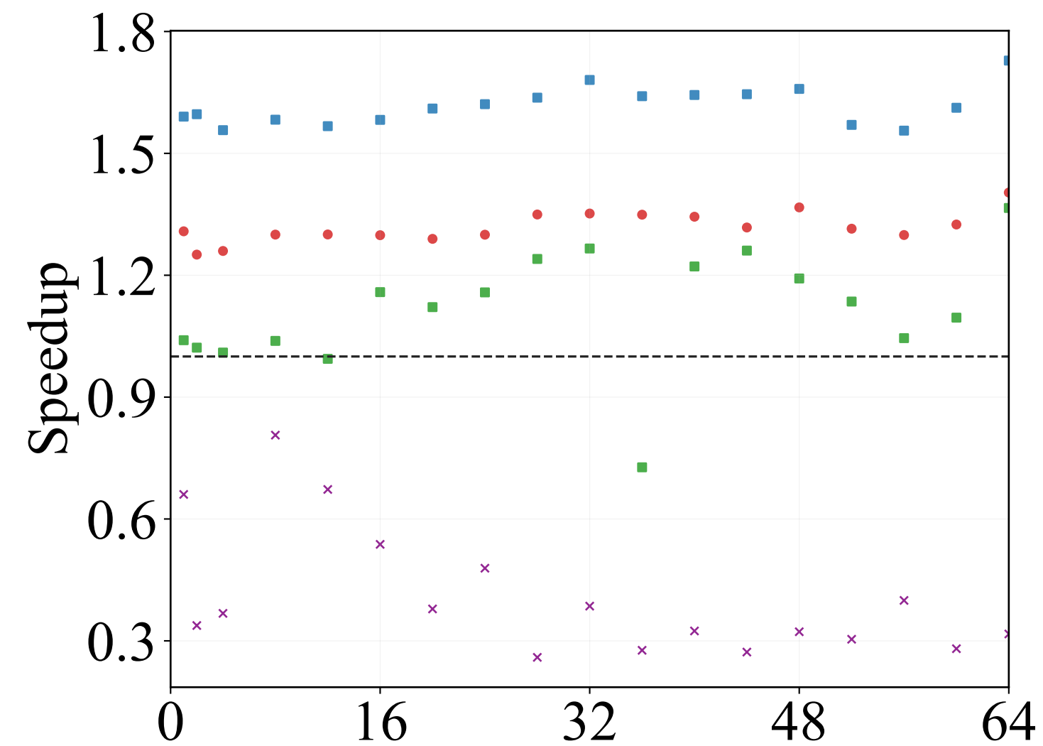
(d) AlexNet on A100
