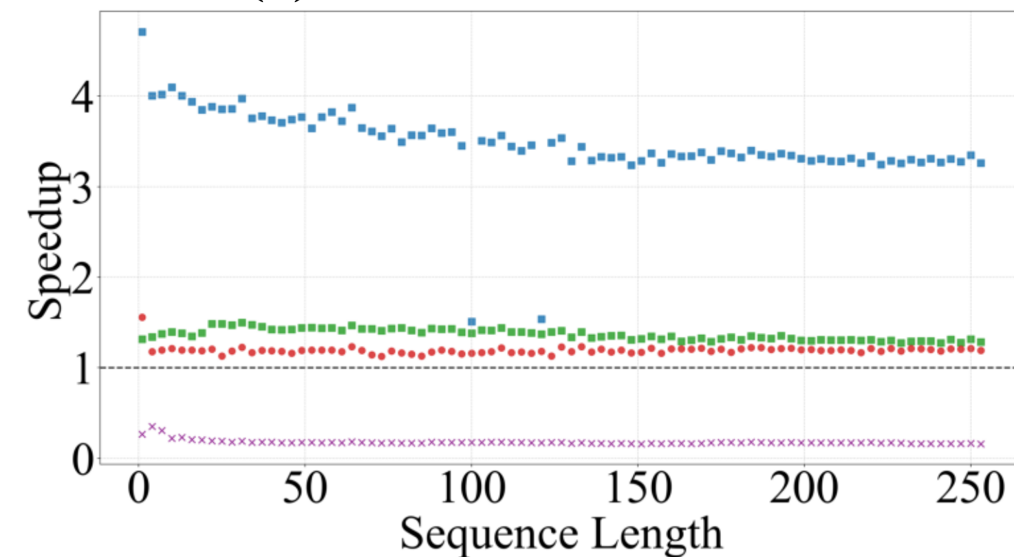
(d) BERT-base on H100
