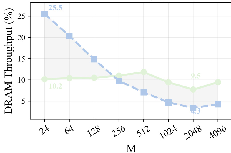
(d) DRAM Throughput (%)
