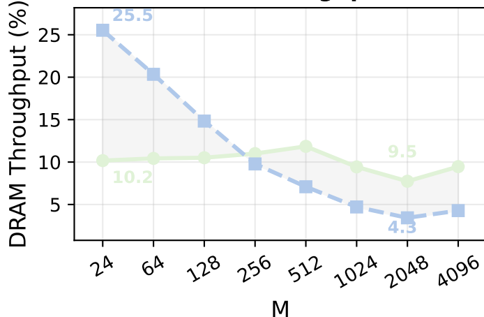
(d) DRAM Throughput (%)
