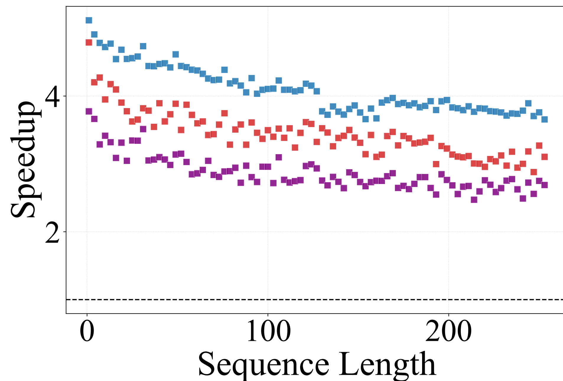
(d) ResNet-101
