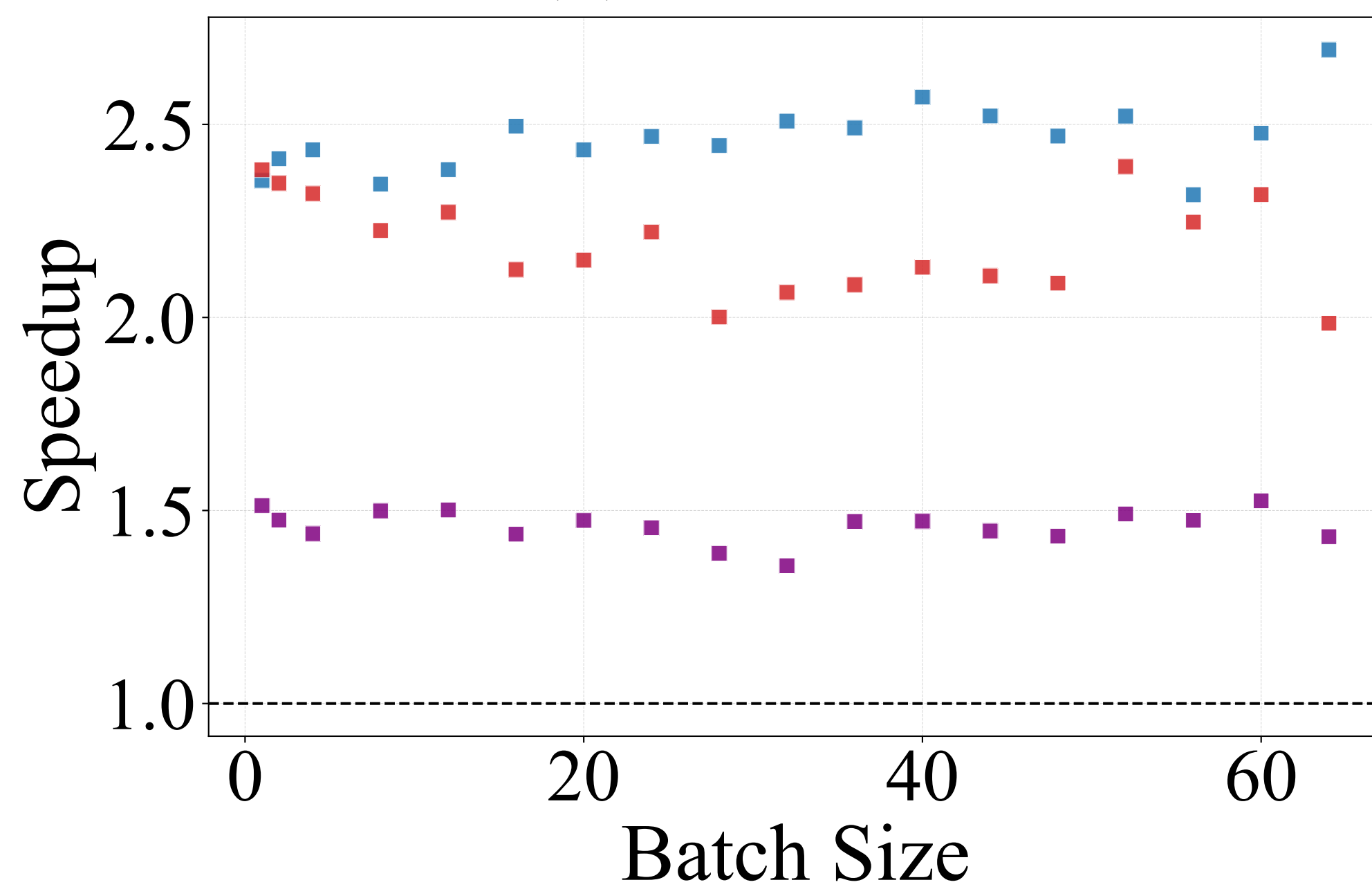
(d) ResNet-101
