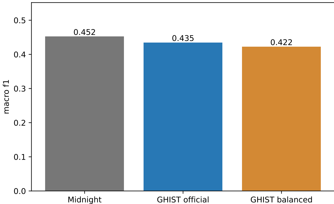
Macro F1
