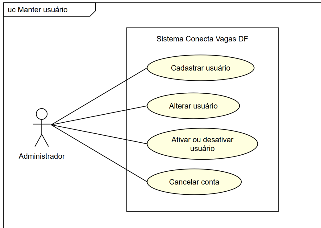
Figura 10 – Diagrama de Caso de Uso Manter Usuário
