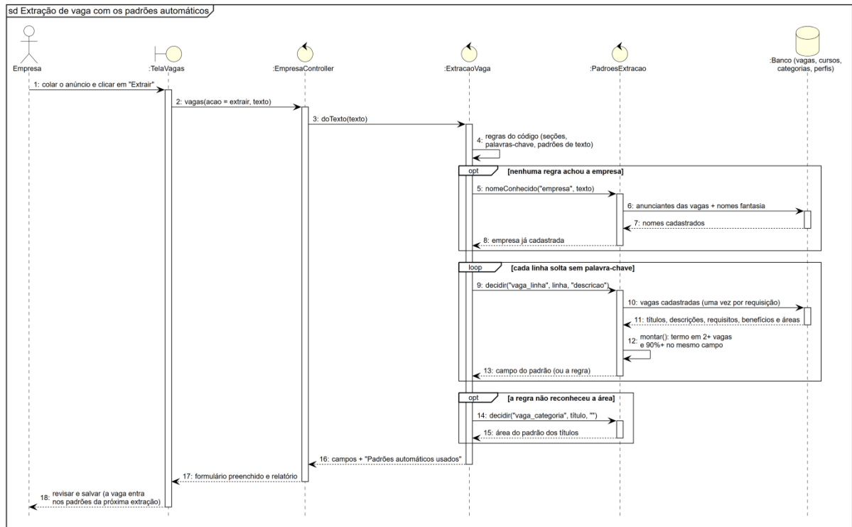
Figura 30 – Diagrama de Sequência Extração de Vaga com os Padrões Automáticos
