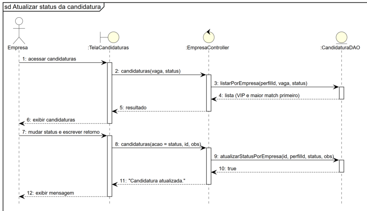
Figura 25 – Diagrama de Sequência Atualizar Status da Candidatura
