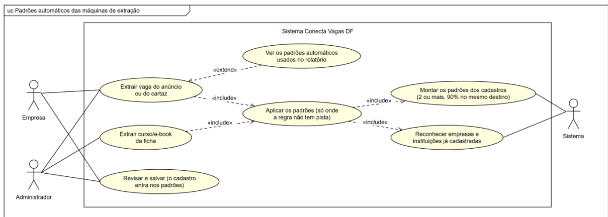
Figura 15 – Diagrama de Caso de Uso Padrões Automáticos da Extração
