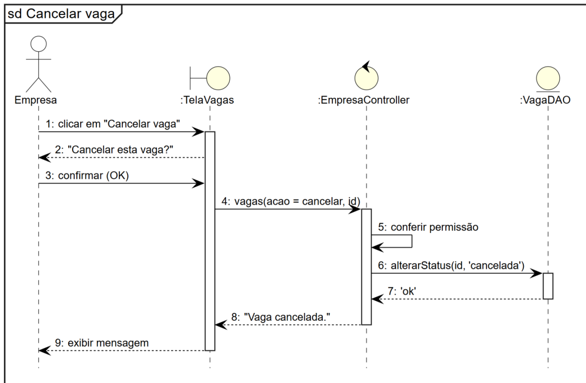
Figura 24 – Diagrama de Sequência Cancelar Vaga
