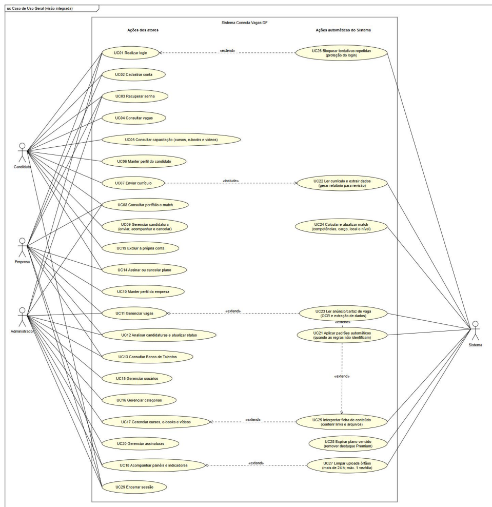
Figura 1 – Diagrama geral de casos de uso do Sistema Conecta Vagas DF
