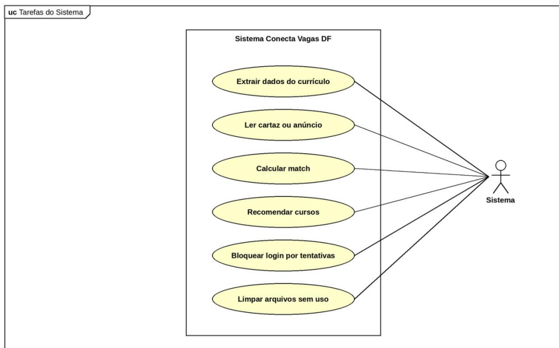
Figura 10 – Diagrama de caso de uso tarefas do sistema
