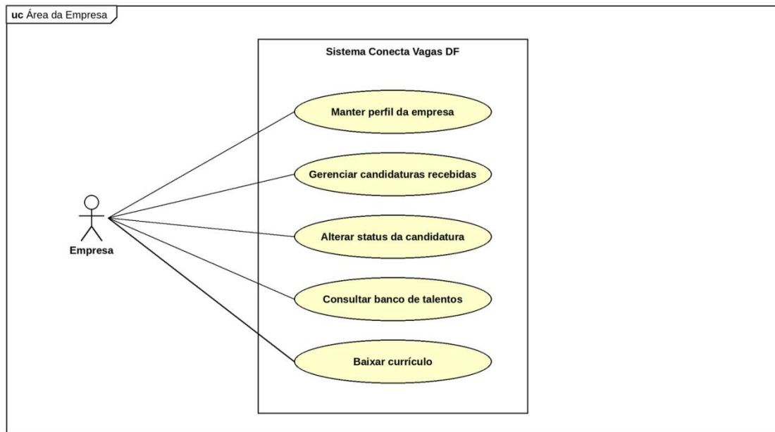
Figura 8 – Diagrama de caso de uso área da empresa
