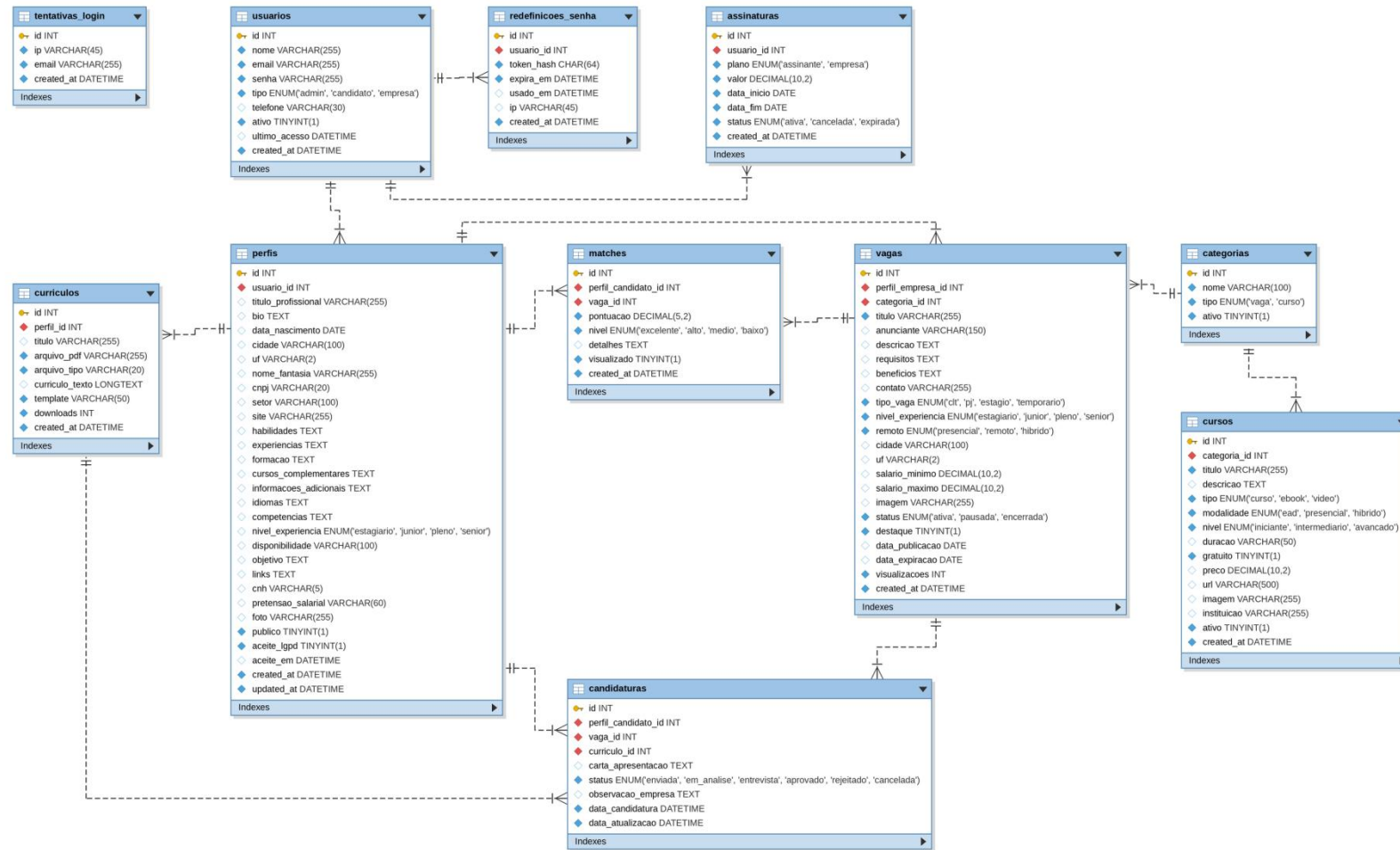
Figura 24 – Diagrama entidade relacionamento do banco tcc_final
