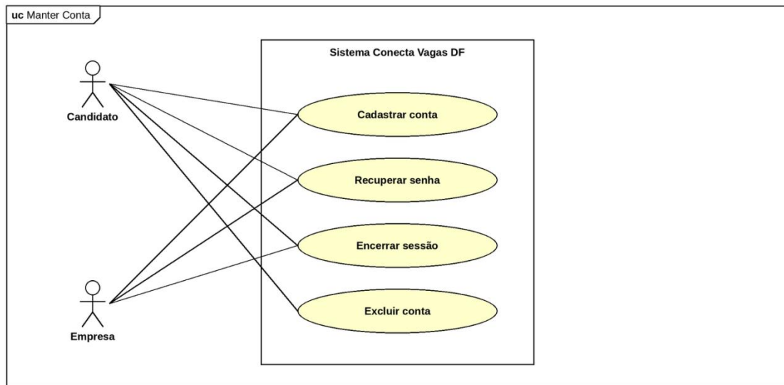
Figura 3 – Diagrama de caso de uso manter conta
