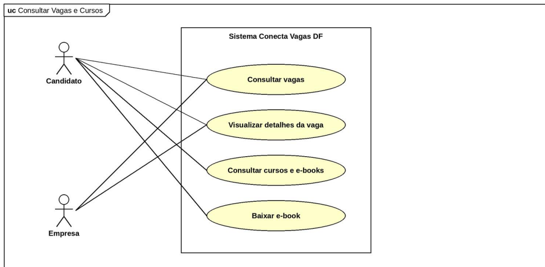
Figura 4 – Diagrama de caso de uso consultar vagas e cursos
