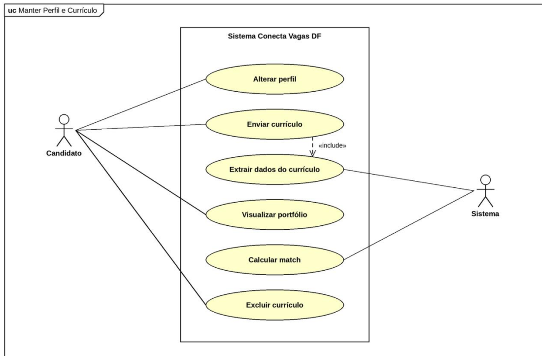
Figura 5 – Diagrama de caso de uso manter perfil e currículo
