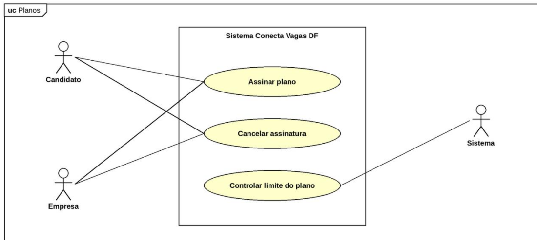
Figura 9 – Diagrama de caso de uso planos
