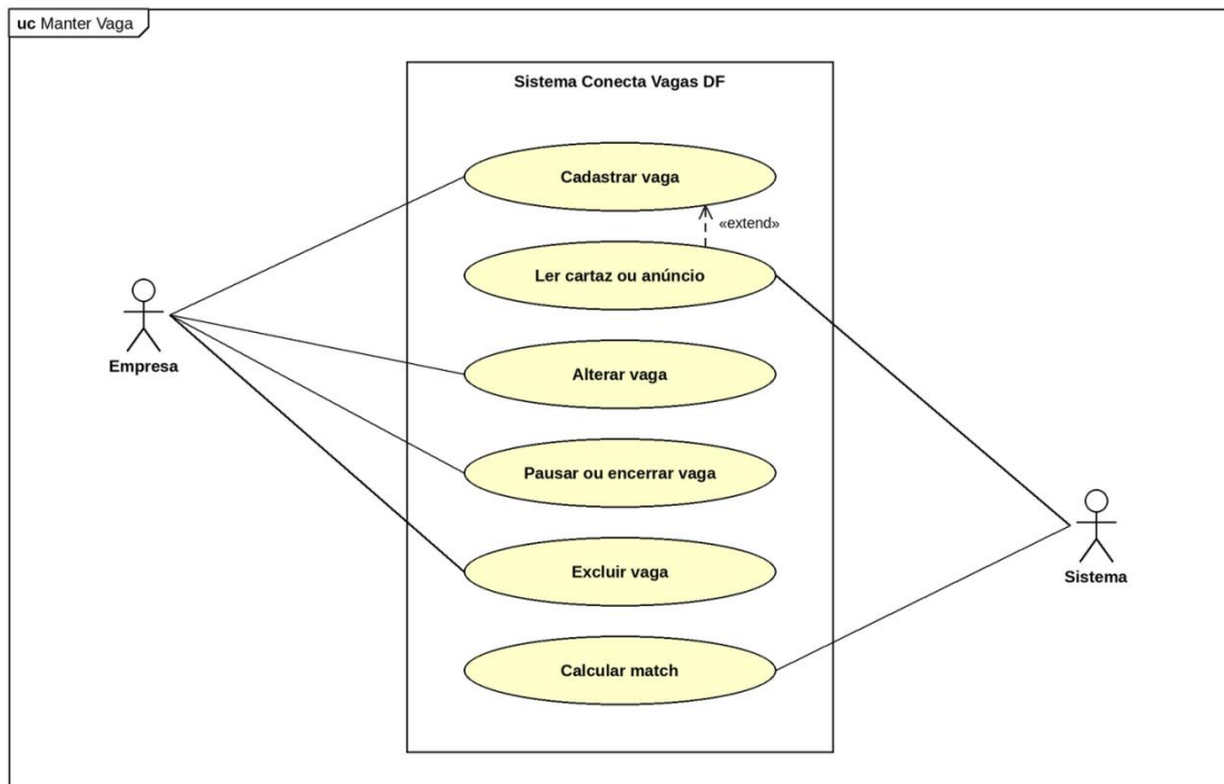
Figura 7 – Diagrama de caso de uso manter vaga
