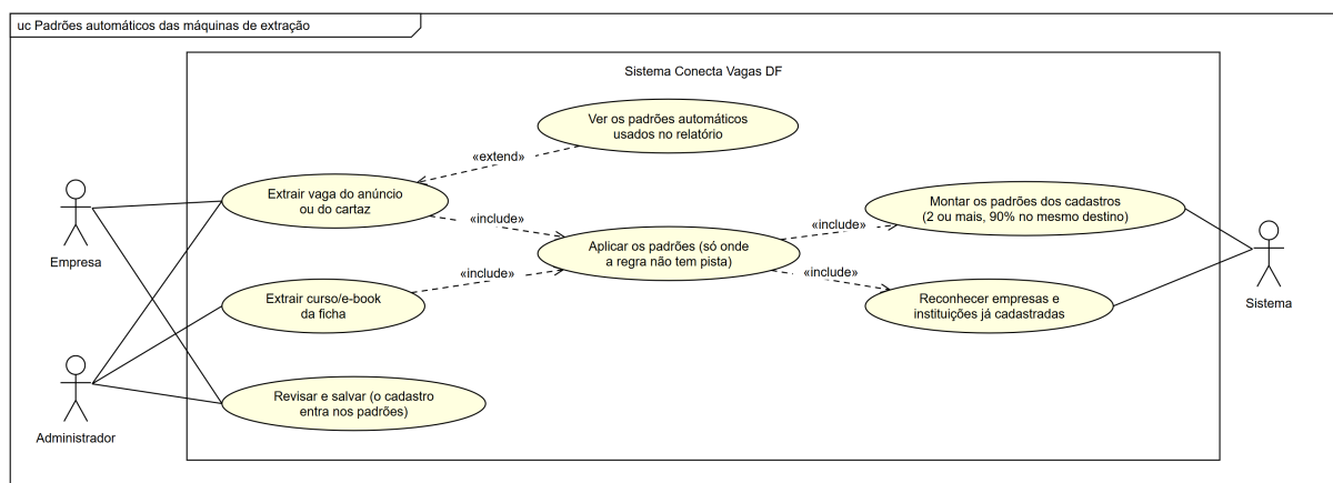
Figura 15 – Diagrama de Caso de Uso Padrões Automáticos da Extração Fonte: Autoria própria (2026).
