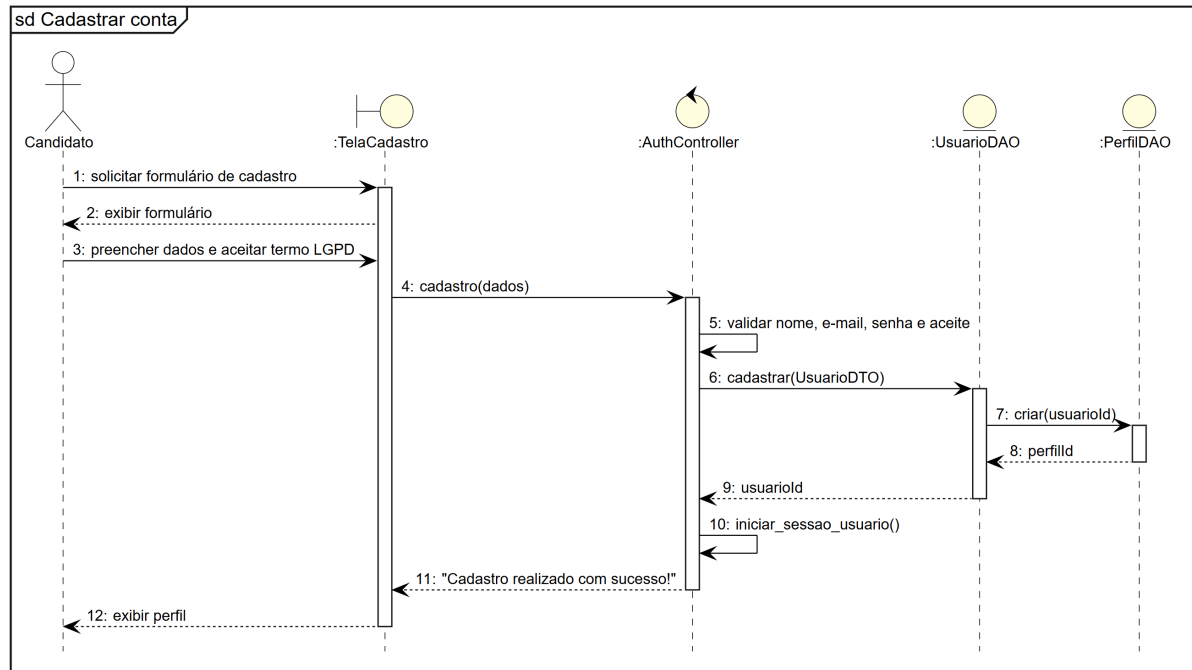
Figura 17 – Diagrama de Sequência Cadastrar Conta Fonte: Autoria própria (2026).
