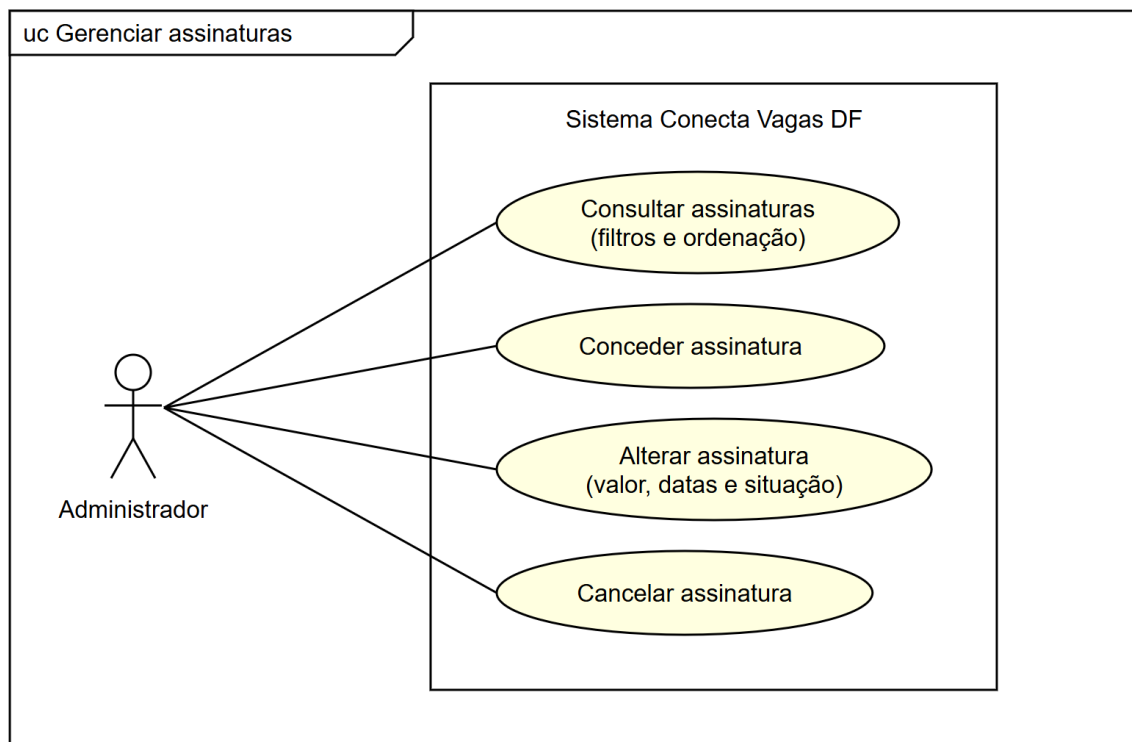
Figura 14 – Diagrama de Caso de Uso Gerenciar Assinaturas Fonte: Autoria própria (2026).
