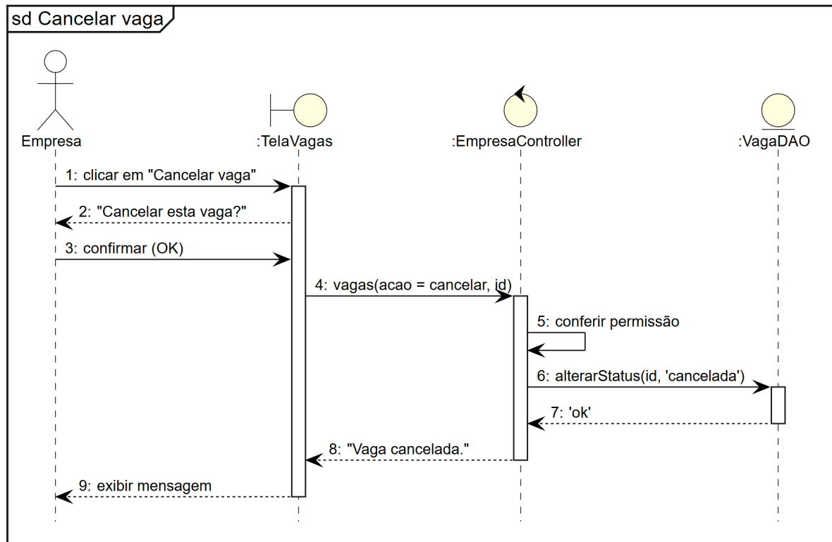
Figura 24 – Diagrama de Sequência Cancelar Vaga Fonte: Autoria própria (2026).
