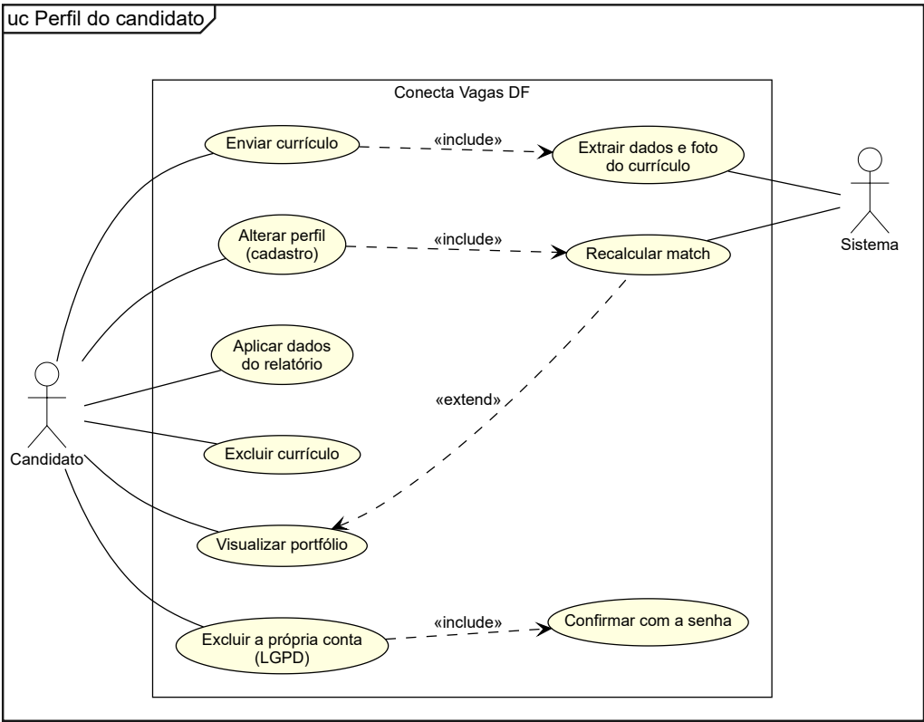
Figura 5 – Caso de uso específico – perfil do candidato
