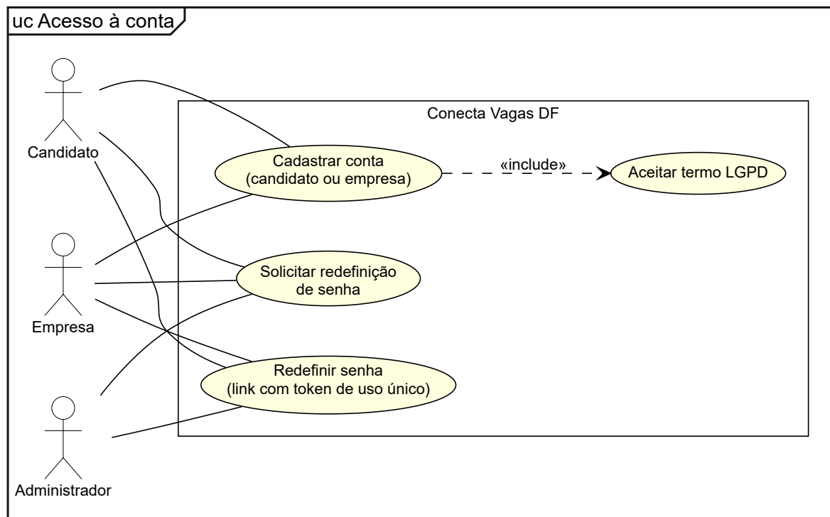
Figura 3 – Caso de uso específico – acesso à conta
