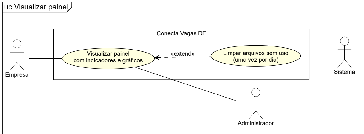
Figura 13 – Caso de uso específico – visualizar painel
