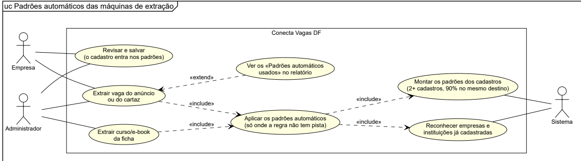
Figura 15 – Caso de uso específico – padrões automáticos da extração
