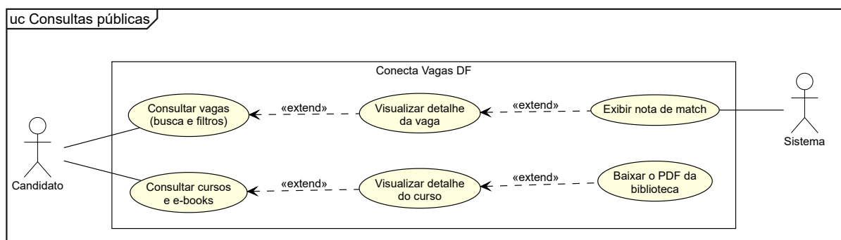
Figura 4 – Caso de uso específico – consultas públicas
