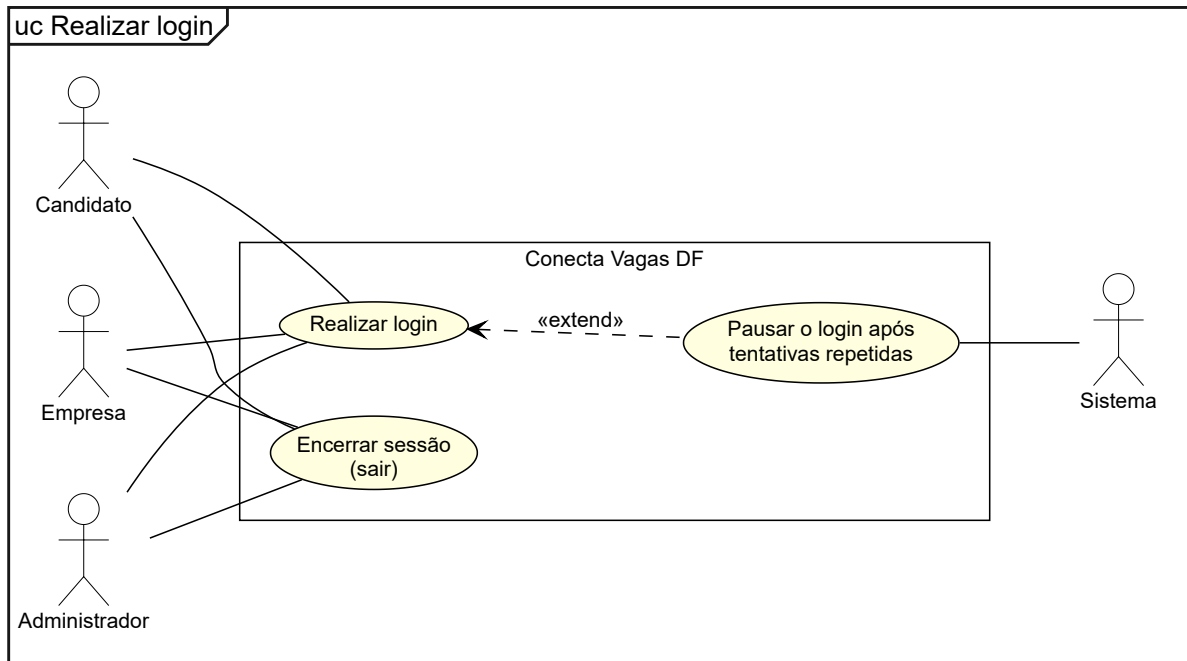
Figura 2 – Caso de uso específico – realizar login
