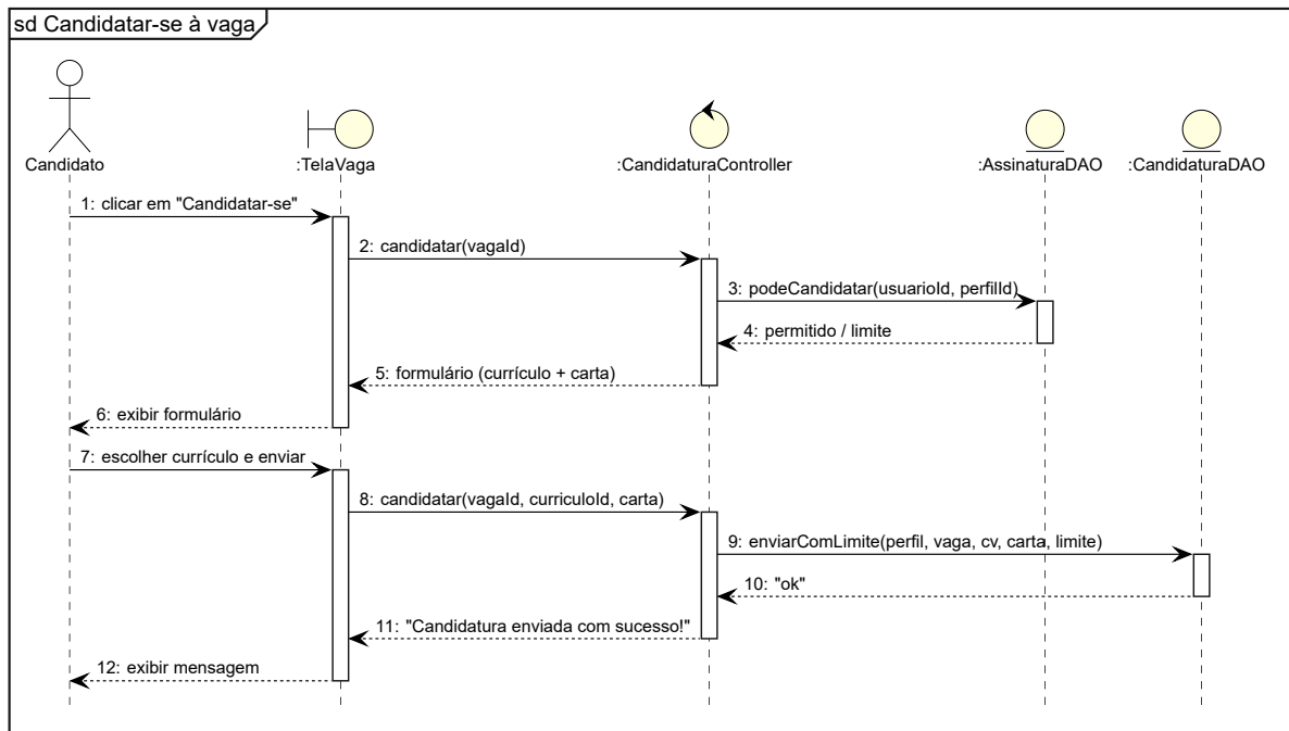
Figura 21 – Diagrama de Sequência candidatar-se à vaga
