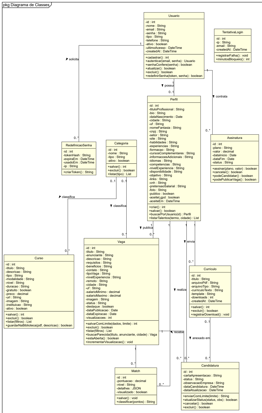
Figura 16 – Diagrama de Classes do domínio
