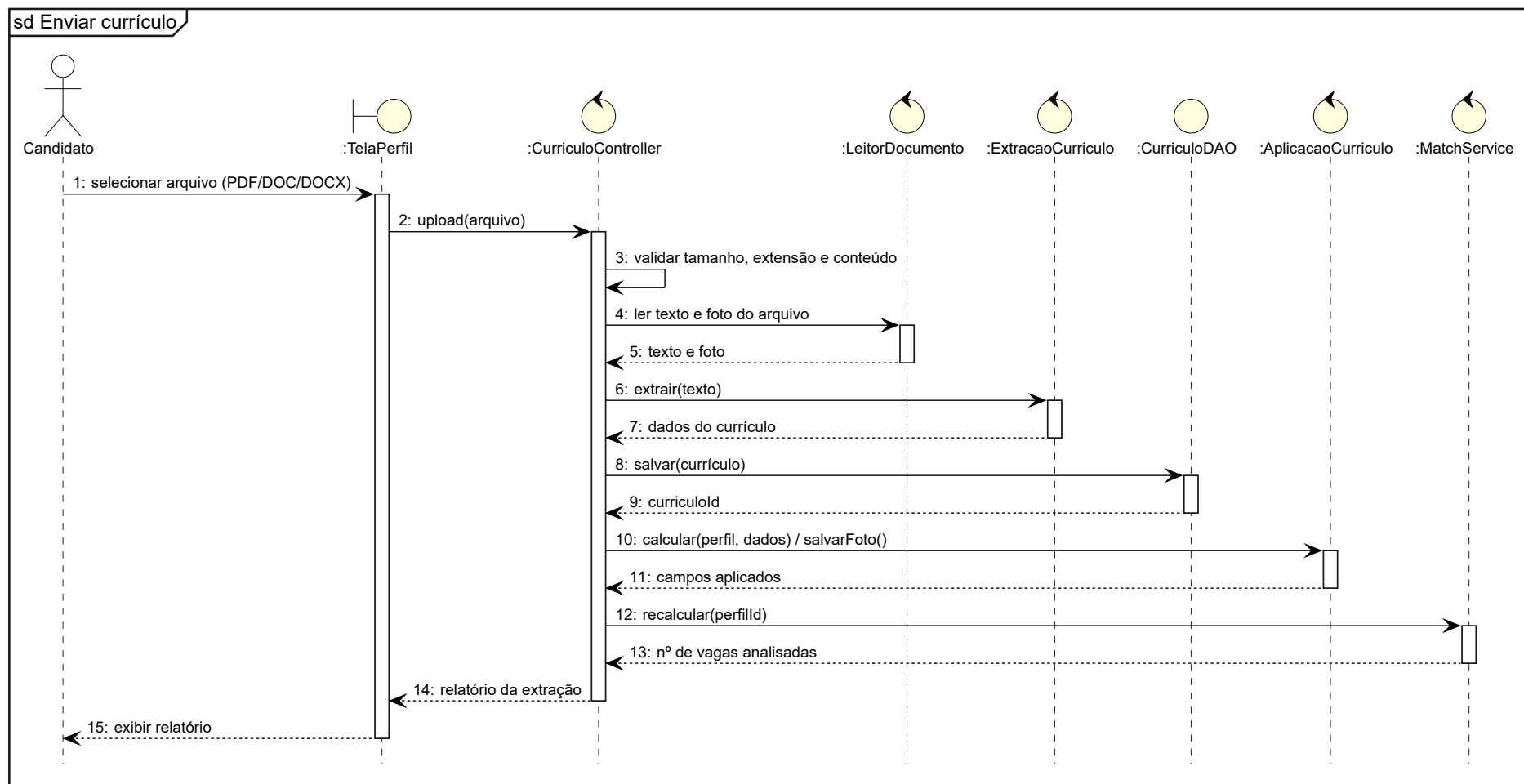
Figura 20 – Diagrama de Sequência enviar currículo (extração e match)
