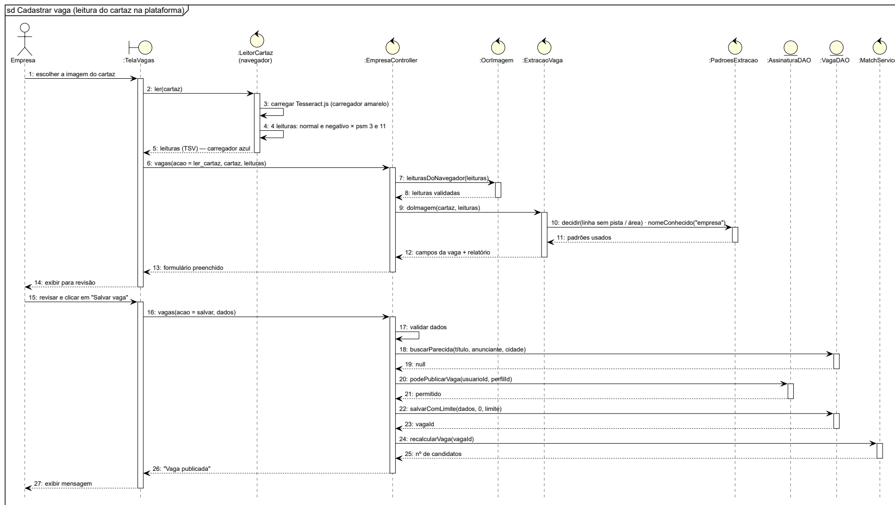
Figura 23 – Diagrama de Sequência cadastrar vaga (leitura do cartaz no navegador e extração)
