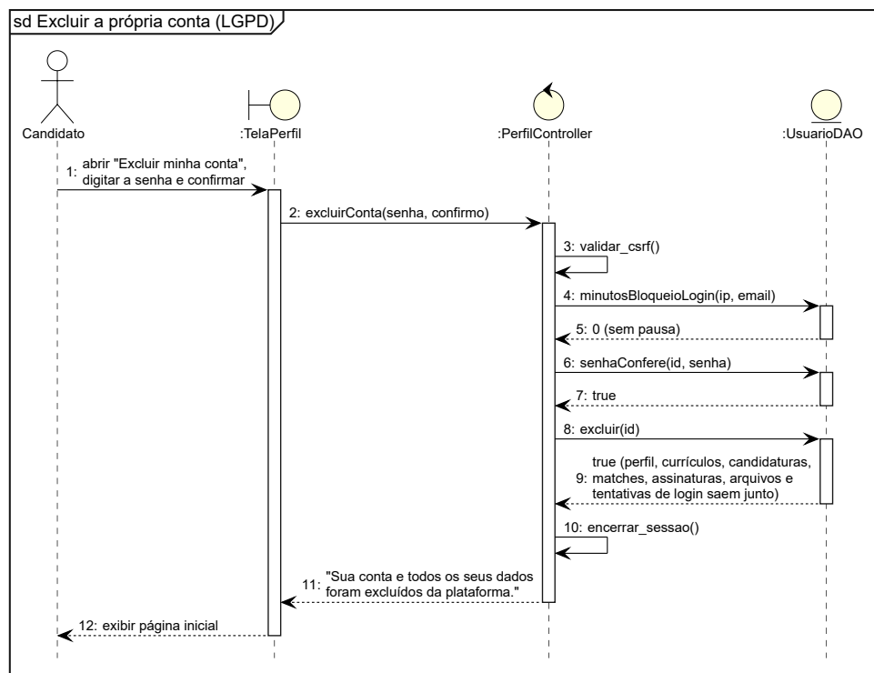
Figura 29 – Diagrama de Sequência excluir a própria conta (LGPD)
