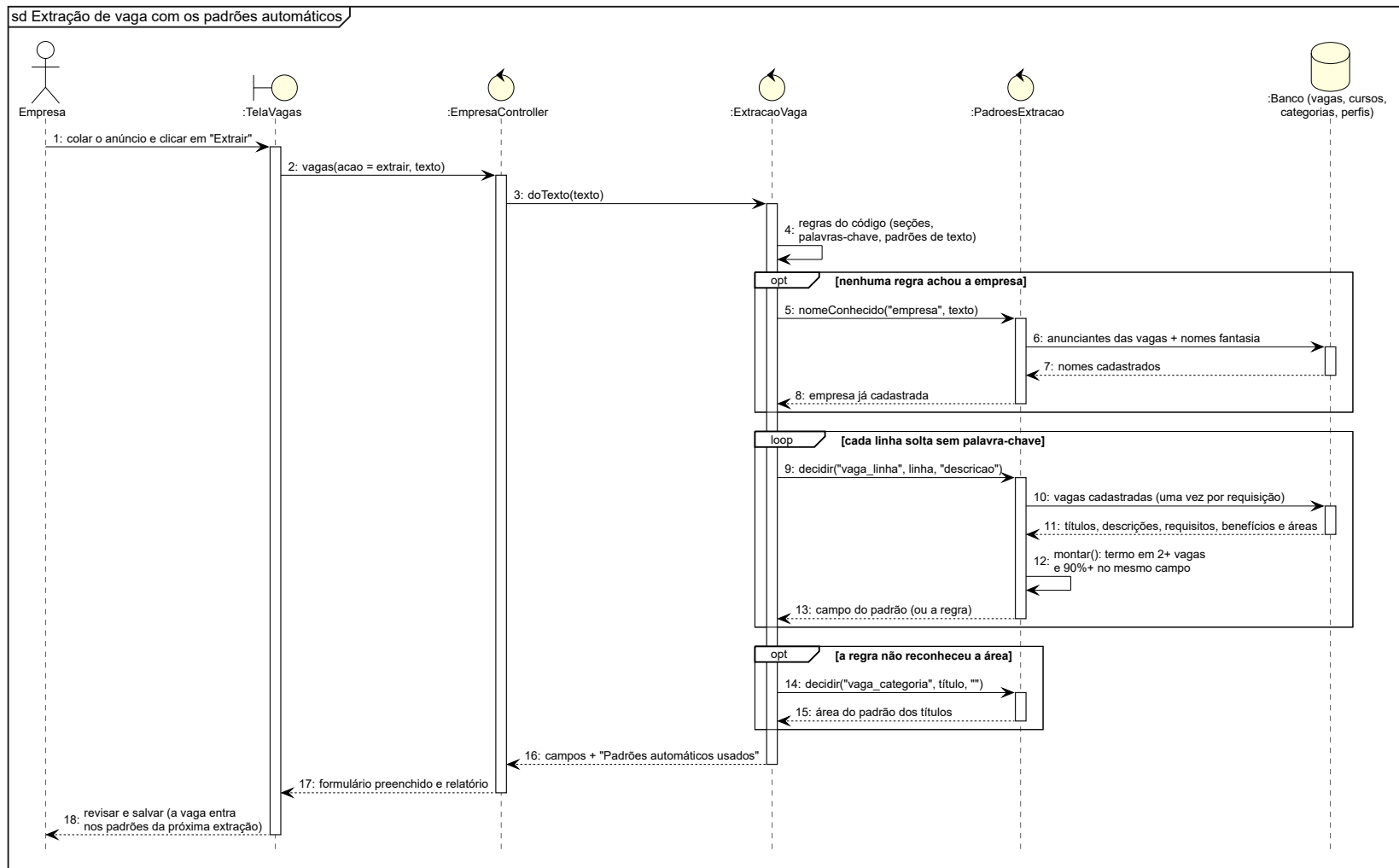
Figura 31 – Diagrama de Sequência extração de vaga com os padrões automáticos
