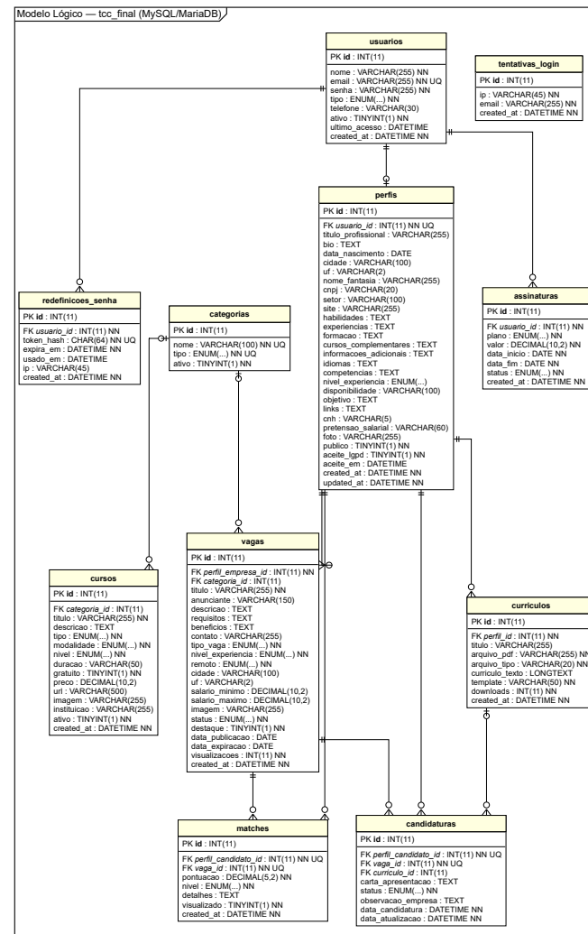
Figura 33 – Modelo Lógico (Diagrama Entidade-Relacionamento)
