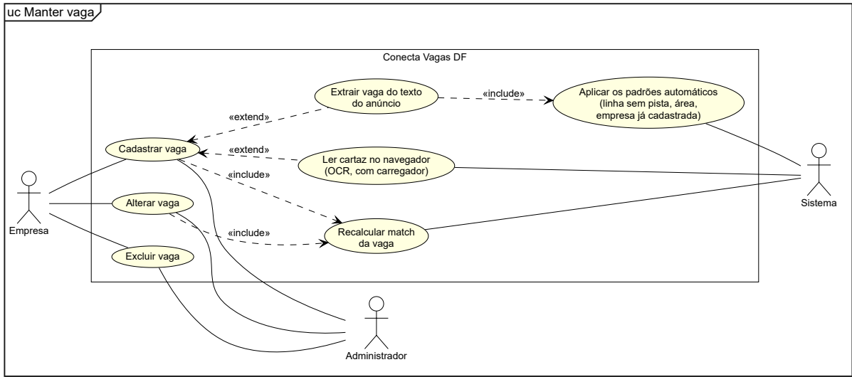
Figura 7 – Caso de uso específico – manter vaga
