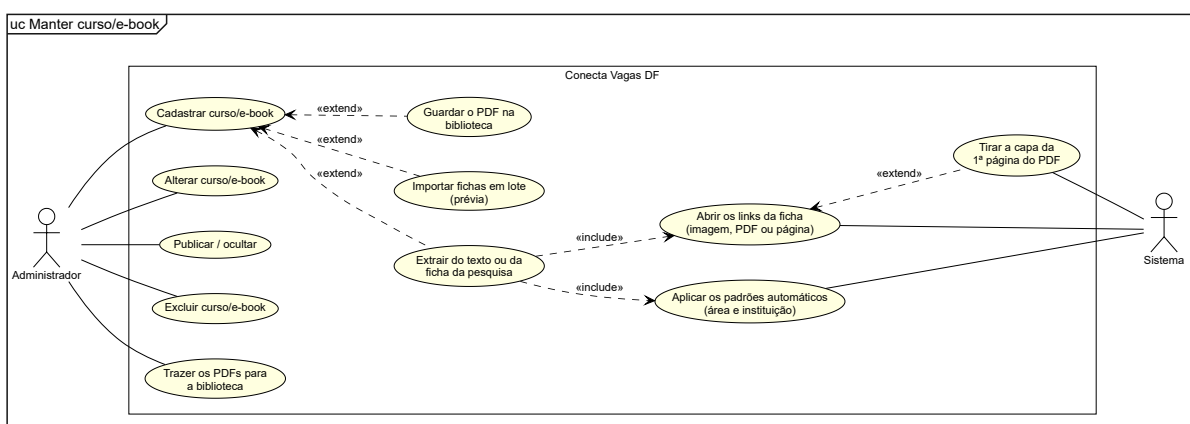
Figura 12 – Caso de uso específico – manter curso/e-book
