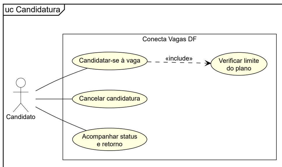
Figura 6 – Caso de uso específico – candidatura
