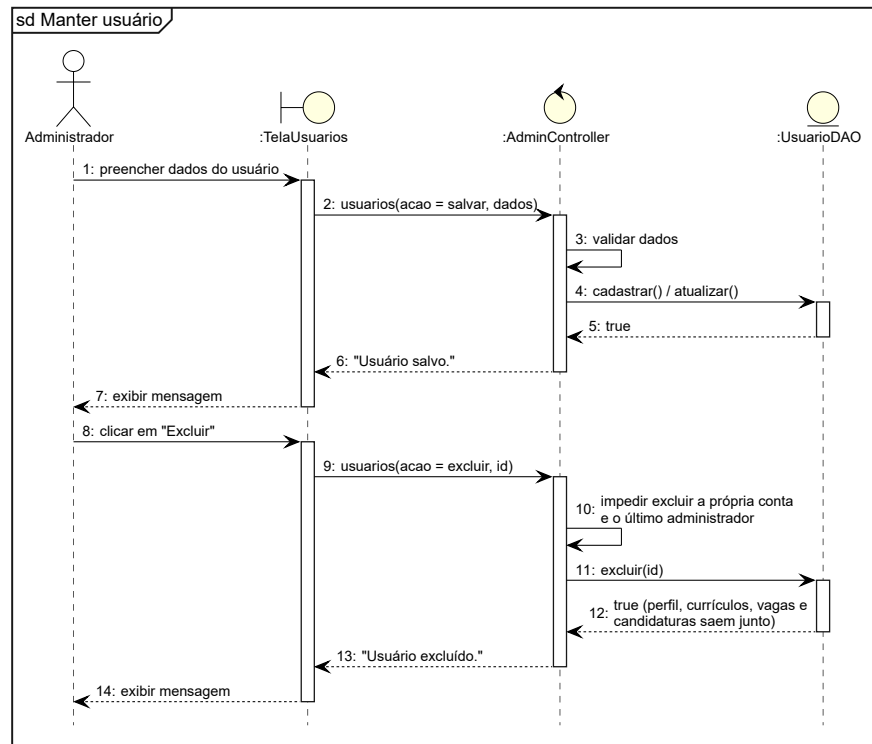
Figura 28 – Diagrama de Sequência manter usuário
