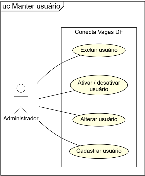
Figura 10 – Caso de uso específico – manter usuário
