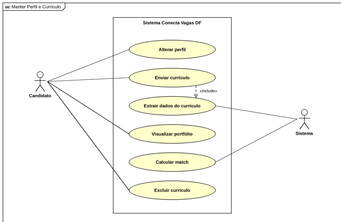
Figura 5 – Diagrama de caso de uso manter perfil e currículo
