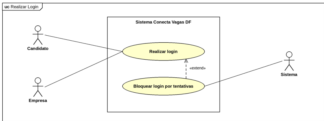
Figura 2 – Diagrama de caso de uso realizar login
