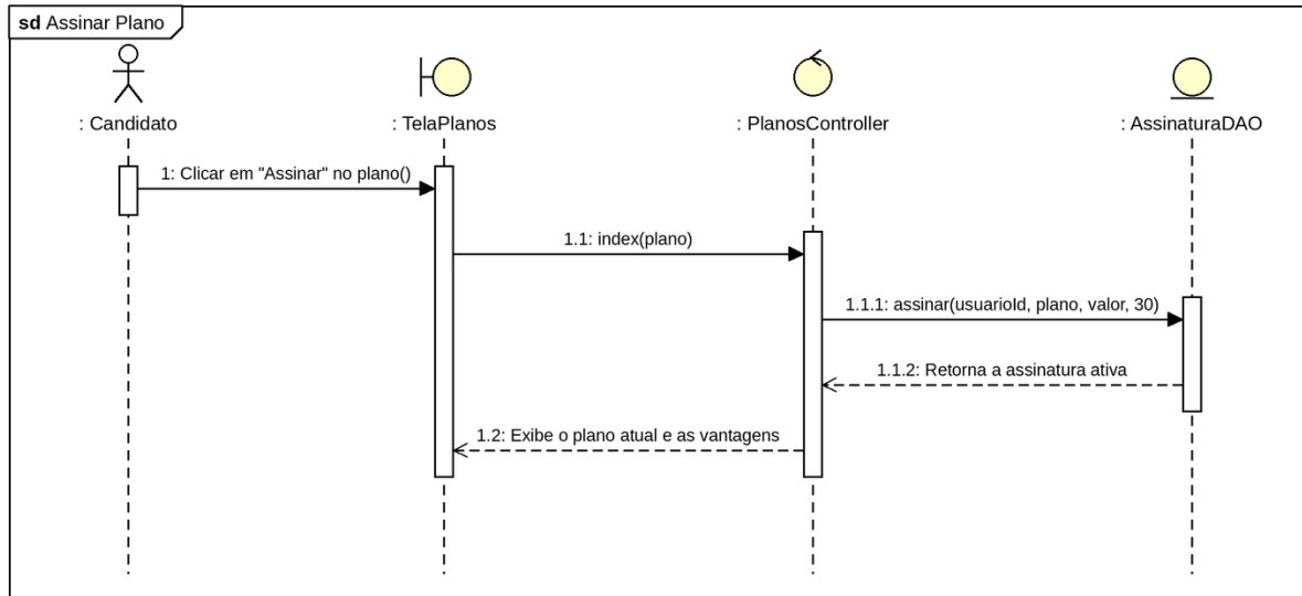
Figura 22 – Diagrama de sequência assinar plano
