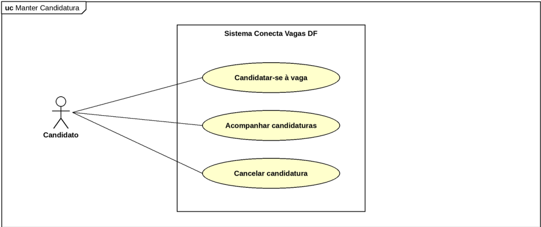
Figura 6 – Diagrama de caso de uso manter candidatura
