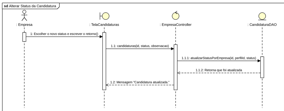
Figura 21 – Diagrama de sequência alterar status da candidatura
