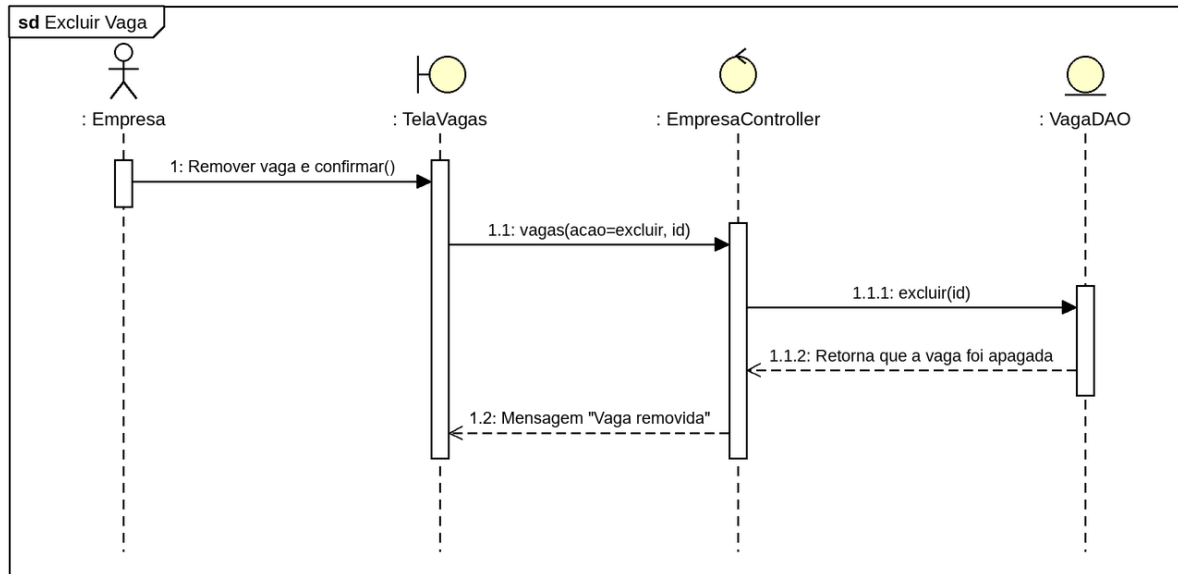
Figura 20 – Diagrama de sequência excluir vaga
