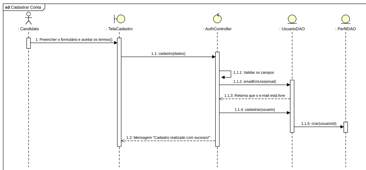
Figura 13 – Diagrama de sequência cadastrar conta
