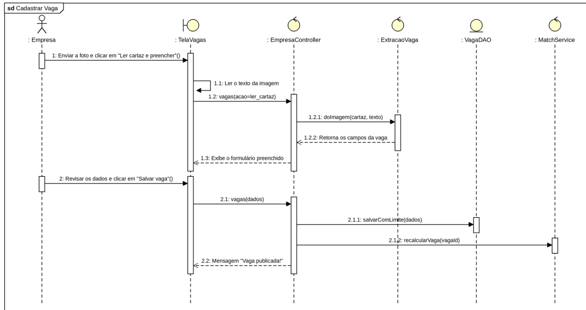
Figura 18 – Diagrama de sequência cadastrar vaga pelo cartaz
