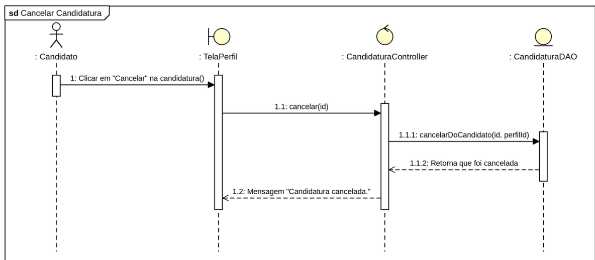
Figura 17 – Diagrama de sequência cancelar candidatura
