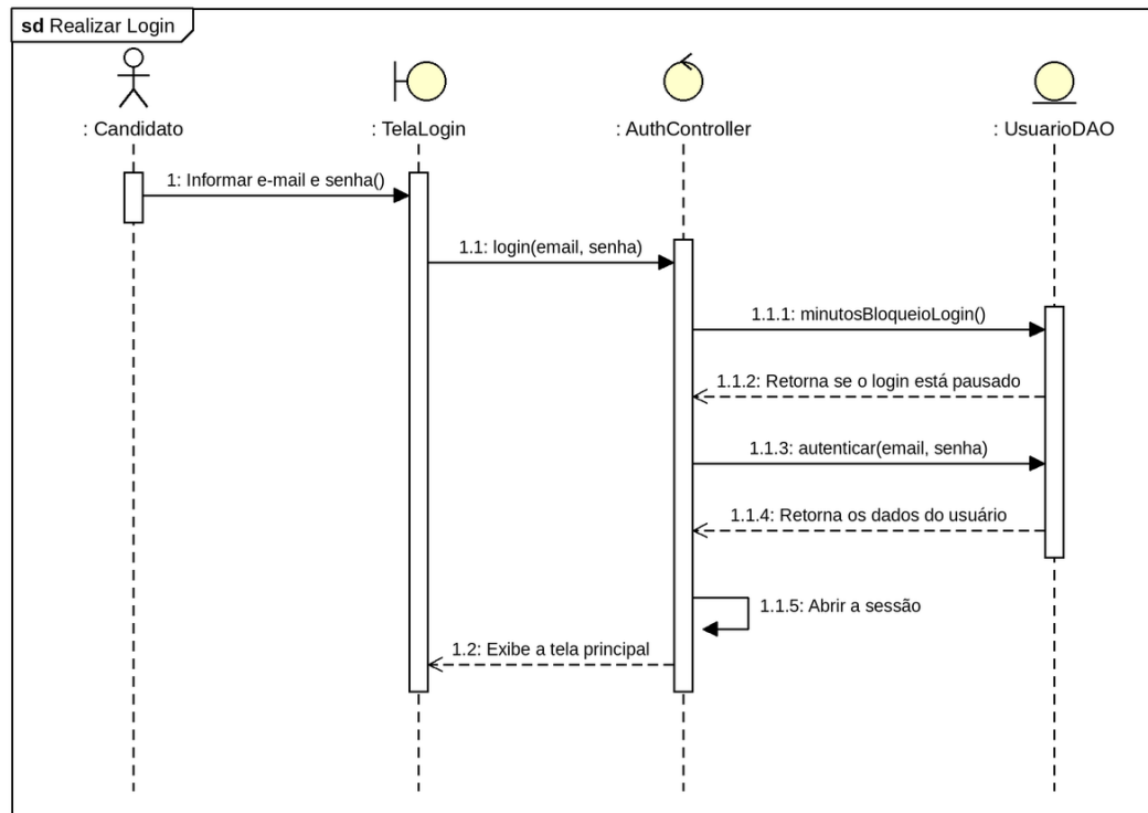
Figura 12 – Diagrama de sequência realizar login
