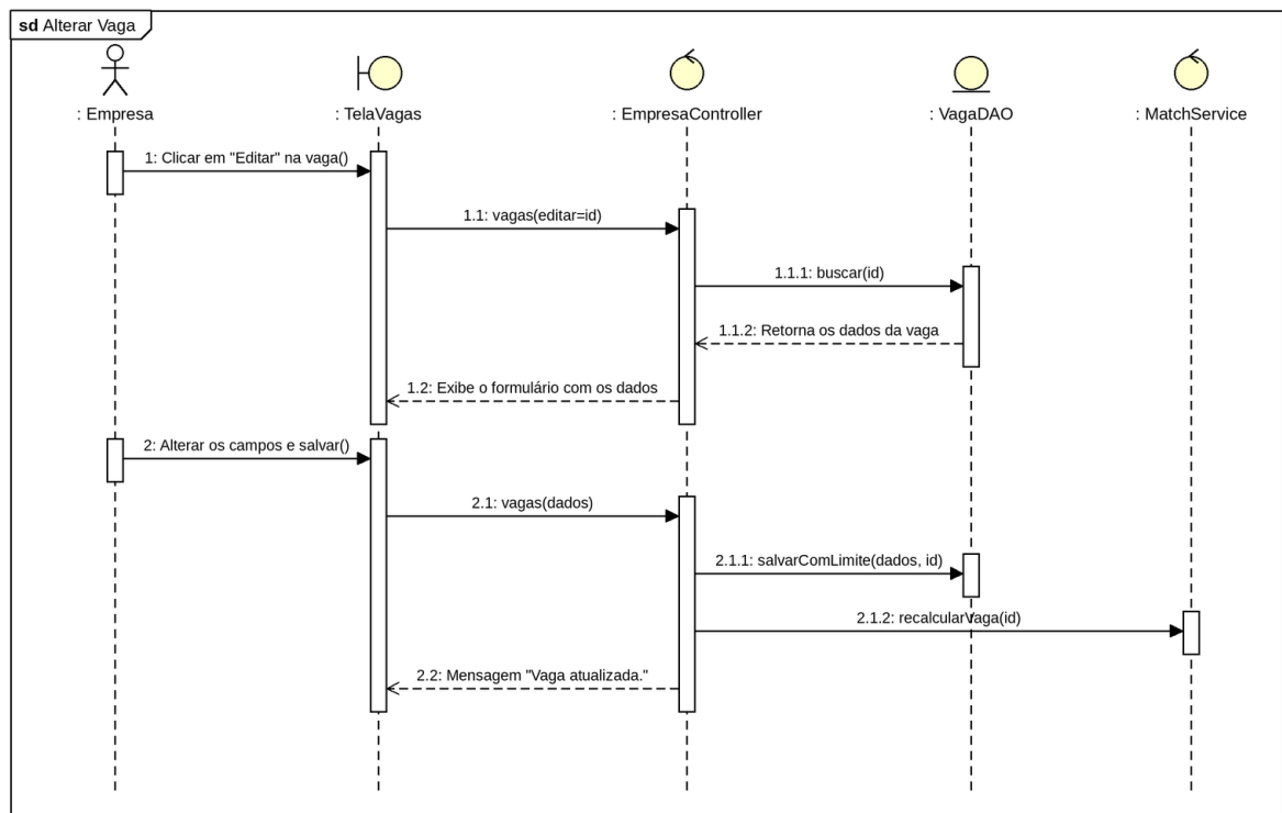
Figura 19 – Diagrama de sequência alterar vaga
