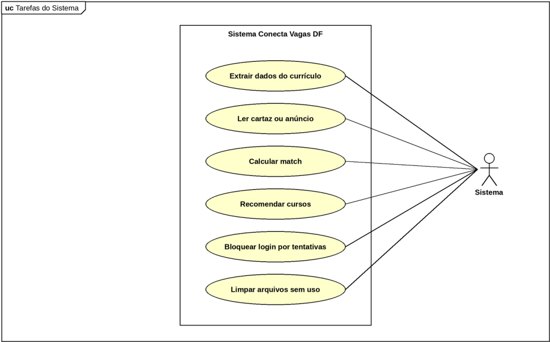
Figura 10 – Diagrama de caso de uso tarefas do sistema
