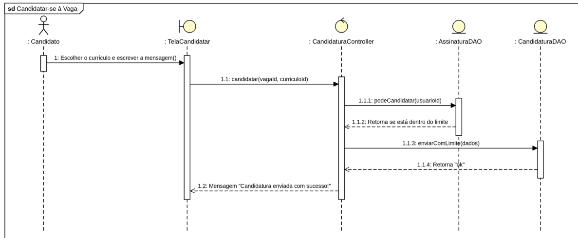
Figura 16 – Diagrama de sequência candidatar-se à vaga
