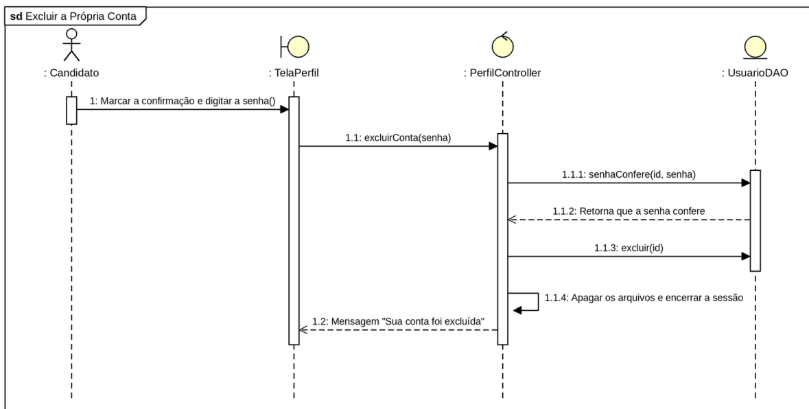
Figura 23 – Diagrama de sequência excluir a própria conta
