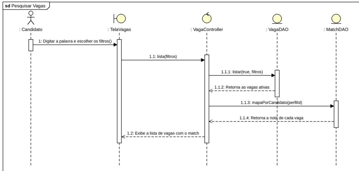
Figura 14 – Diagrama de sequência pesquisar vagas
