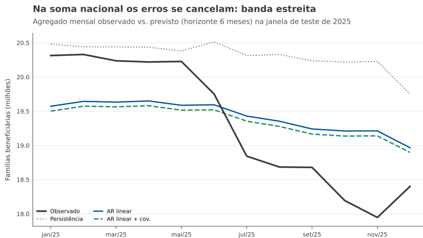
Figura 19 – Ajuste nacional na janela de teste ( H = 6 ). A soma das previsões municipais reproduz o agregado observado de 2025 com erro pequeno; os erros municipais cancelam-se na agregação, o que justifica usar o MAPE nacional como banda da projeção.
