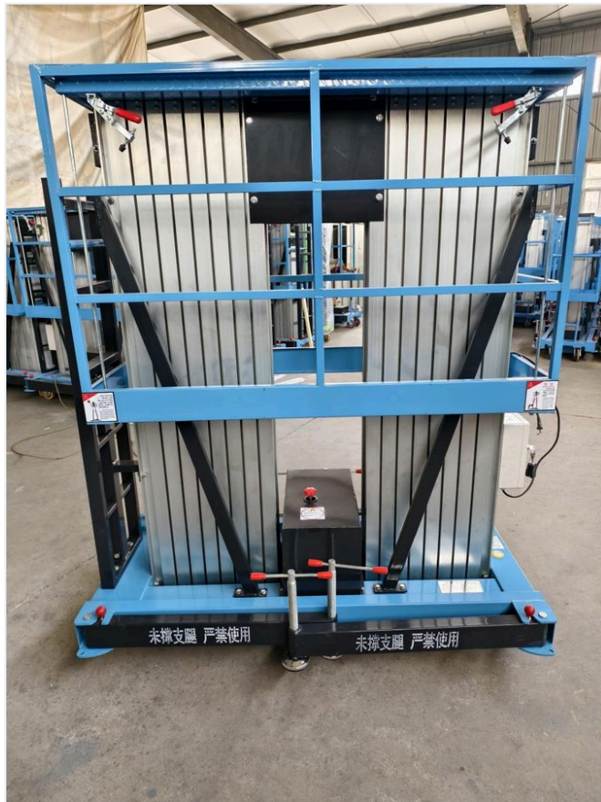
Foto real de la unidad SJYL0.22-12 — mástil de aluminio doble, chasis con ruedas y estabilizadores manuales.
