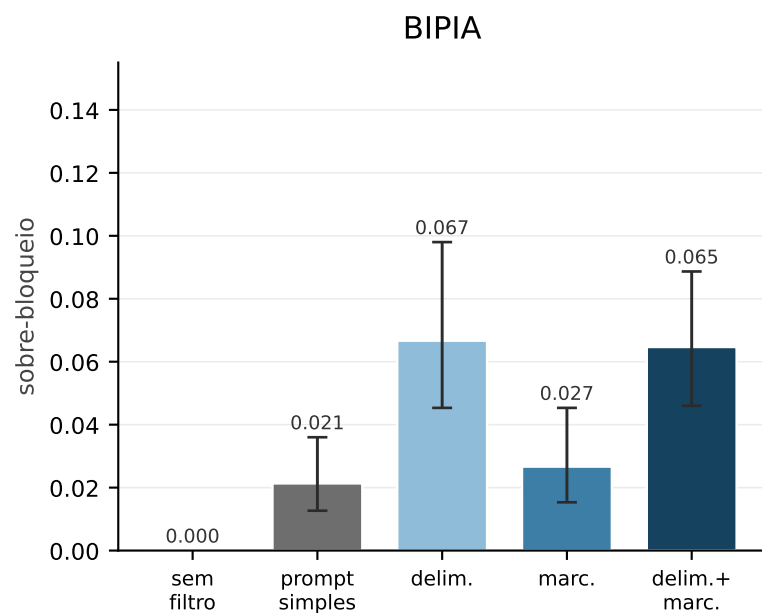
llama-3.1-8b
