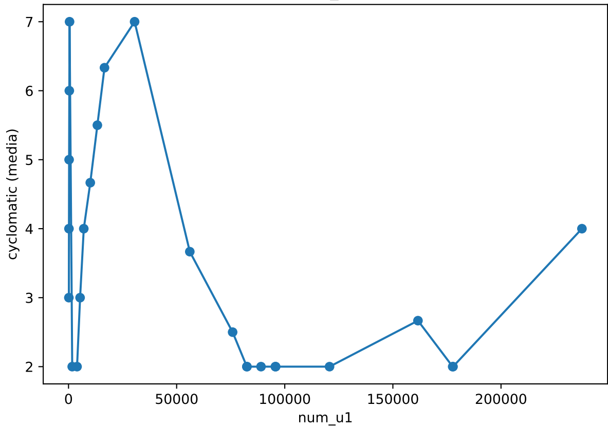
cyclomatic vs num_u1 (media su lr)
