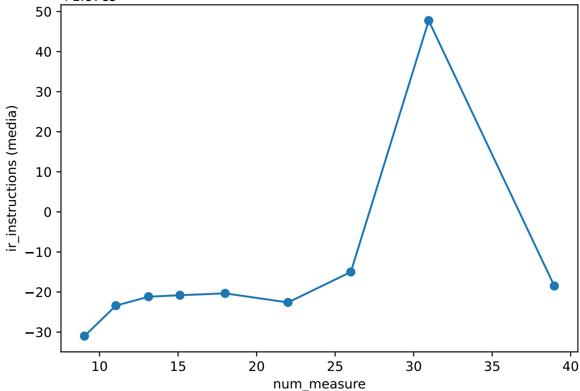
ir_instructions vs num_measure (media su ciclomatic)
