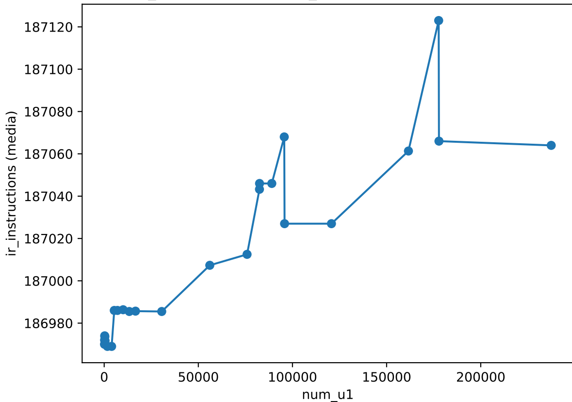
ir_instructions vs num_u1 (media su ciclomatic)
