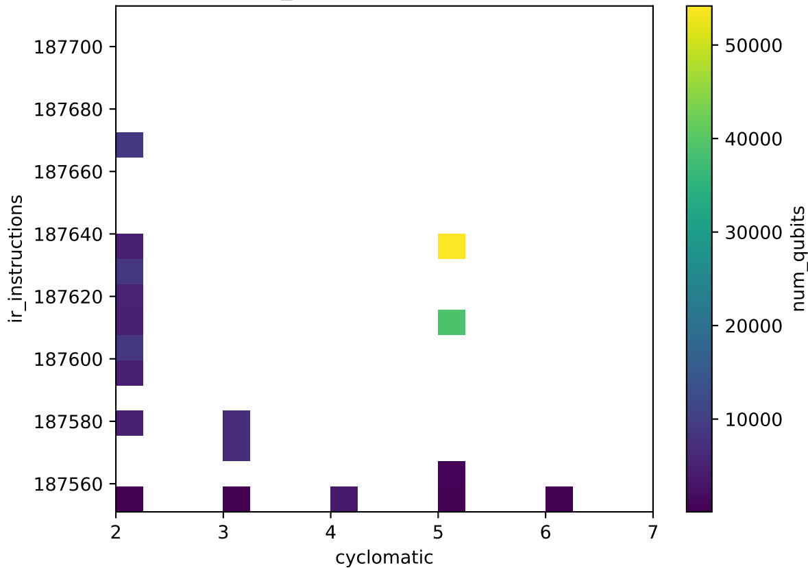
num_qubits (media per bin)
