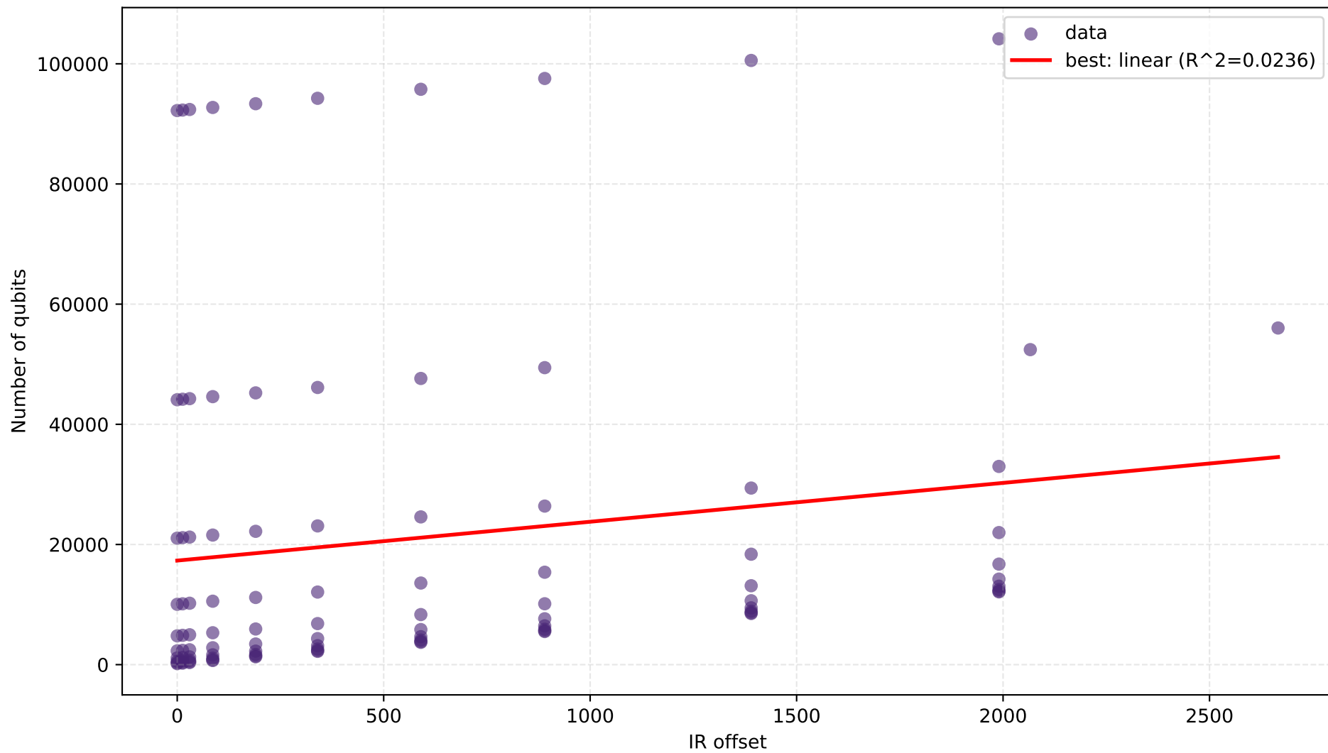
Qubit count vs IR offset
