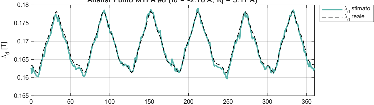
Analisi Punto MTPA #8 ( I_d = -2.76 A, I_q = 3.17 A)
