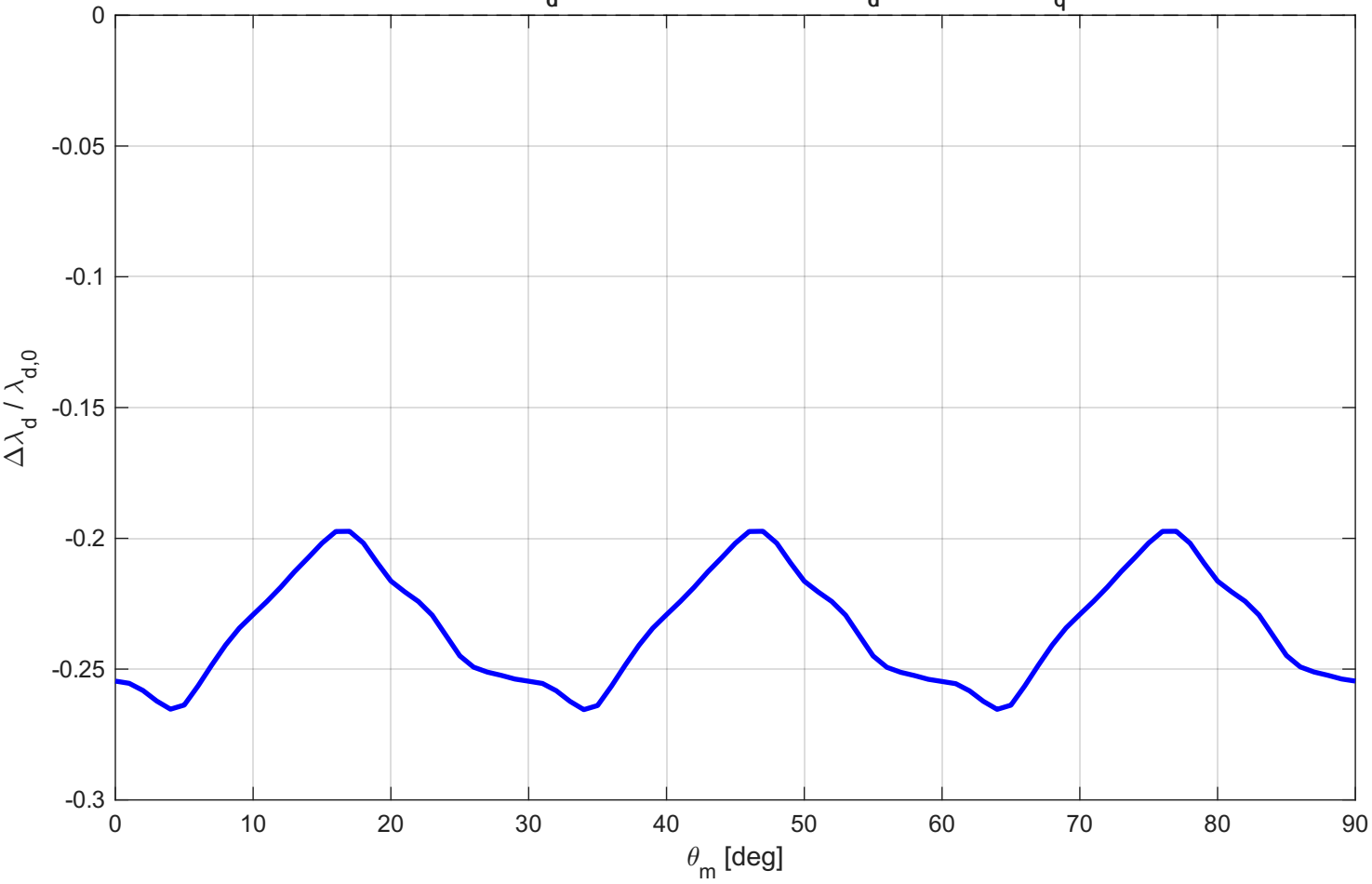
Variazione relativa \lambda_d : MTPA vs A Vuoto (@ i_d = -2.755 A, i_q = 3.17 A)
