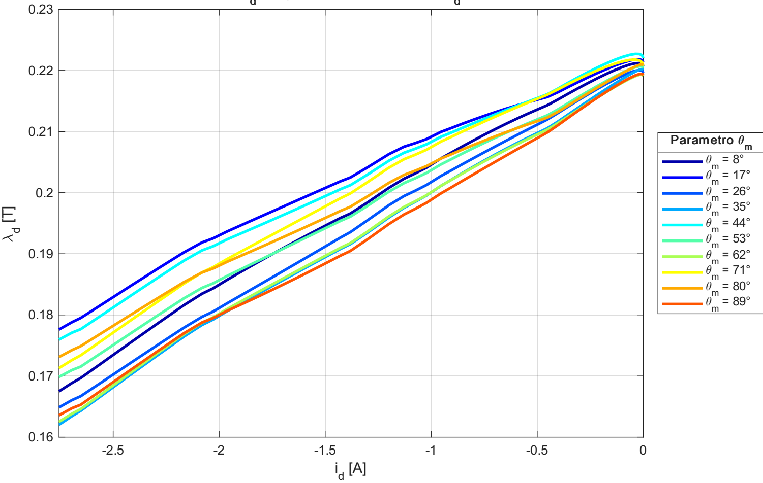
\lambda_d lungo traiettoria MTPA vs i_d
