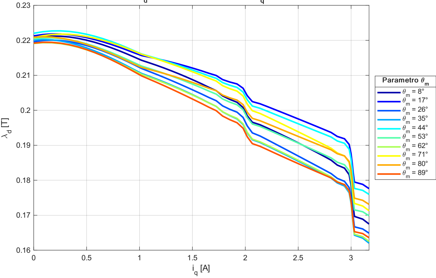
\lambda_d lungo traiettoria MTPA vs i_q
