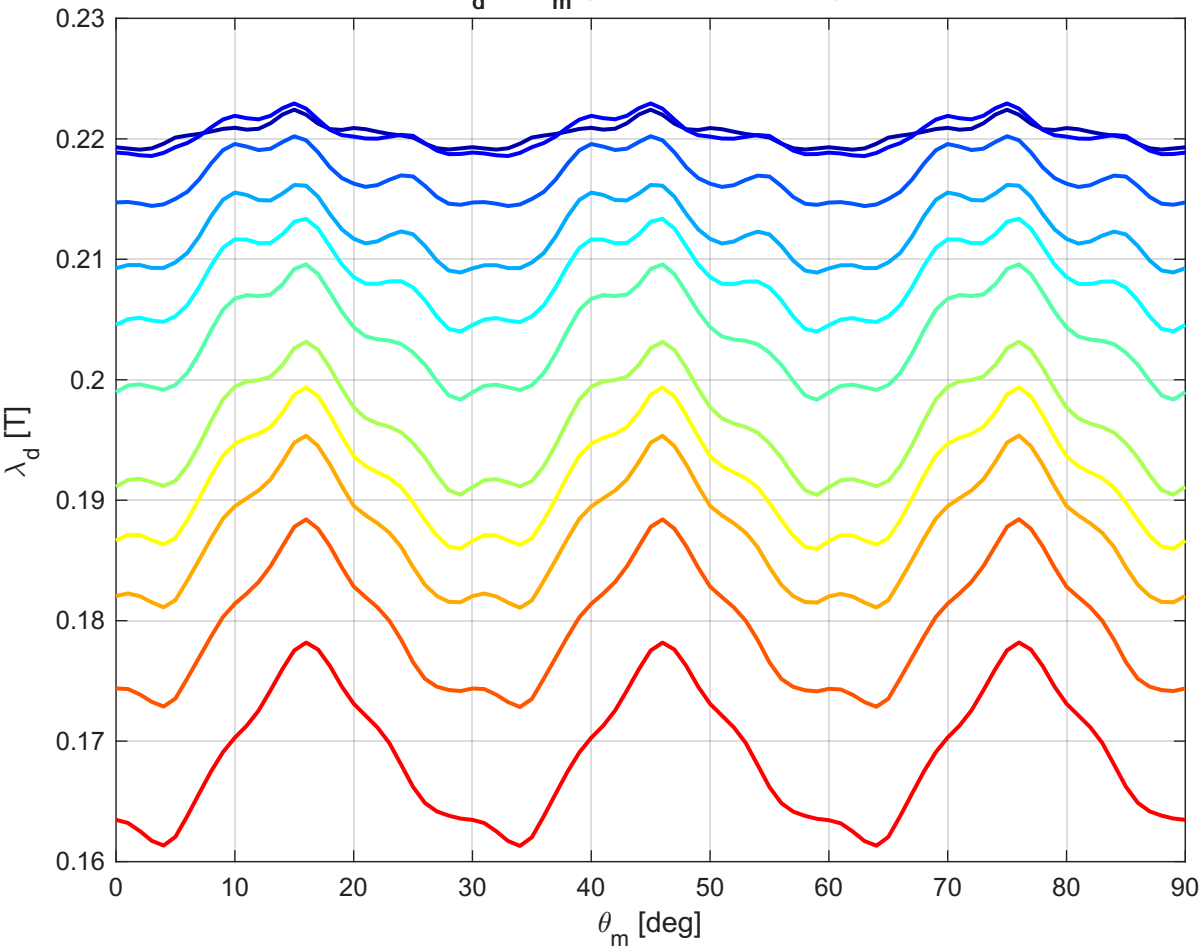
\lambda_d vs \theta_m (Traiettorie MTPA)
