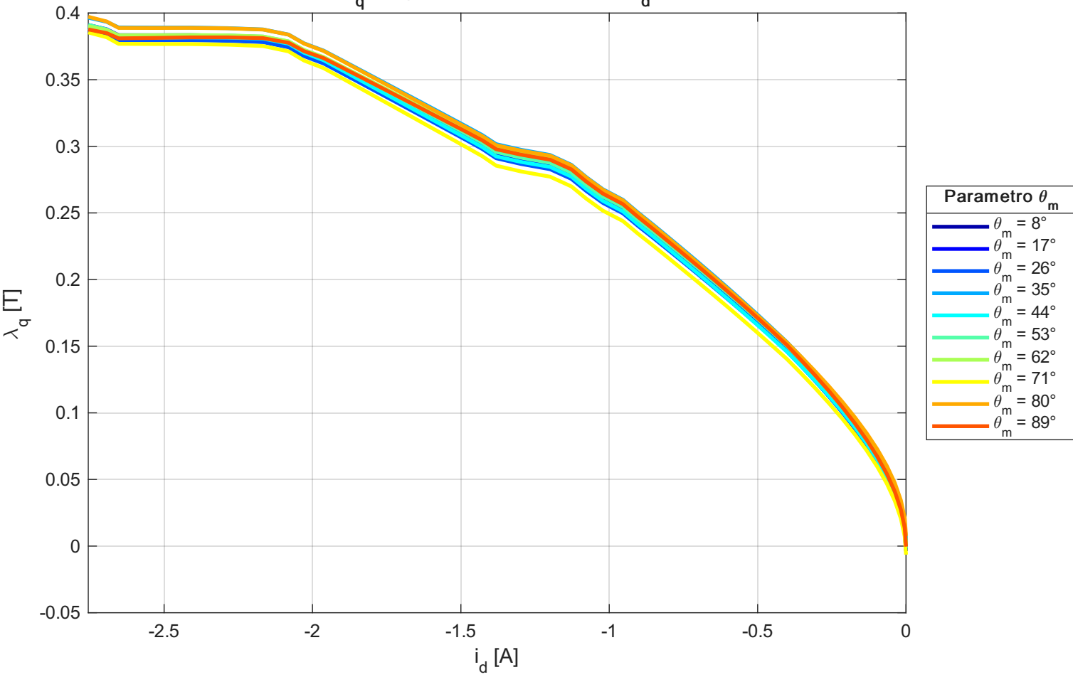
\lambda_q lungo traiettoria MTPA vs i_d
