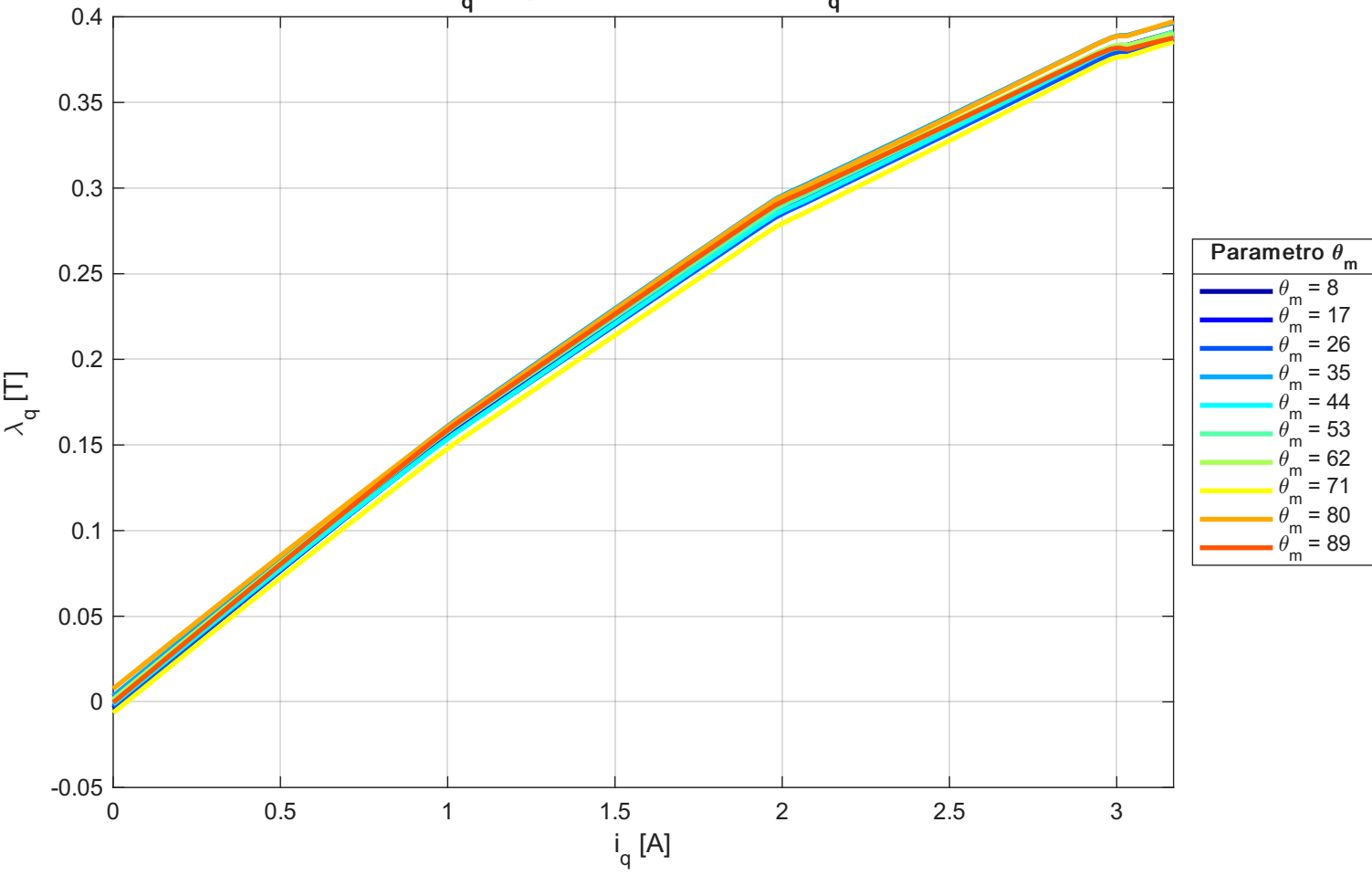
\lambda_q lungo traiettoria MTPA vs i_q
